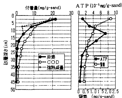
図-5 砂への付着量の変化
