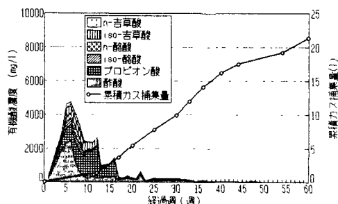
図-3 有機酸の構成と累積ガス捕集量（植種カラム）
