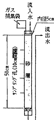
図-1 実験装置
