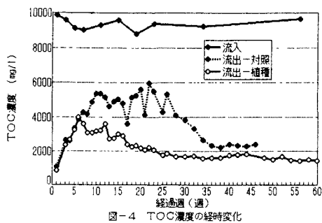
図-4 TOC濃度の経時変化
