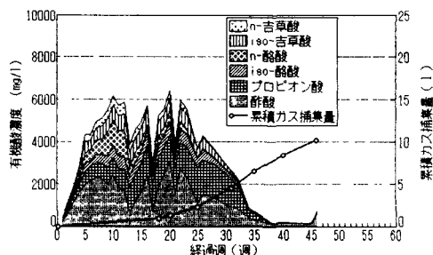
図-2 有機酸の構成と累積ガス捕集量（対照カラム）
