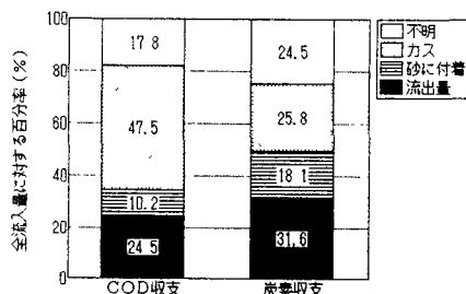
図-6 COD・炭素収支
