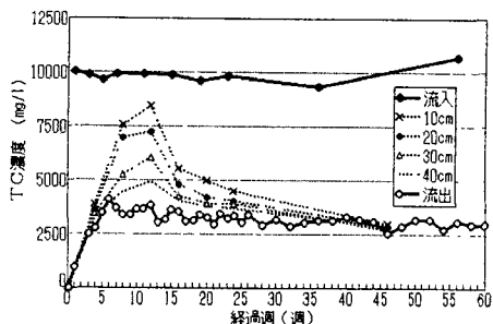
図-7 深さごとのTCの変化
