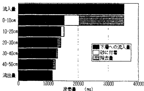
図-8 深さごとの炭素収支
