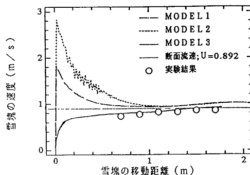
図-4 雪塊の速度の比較
