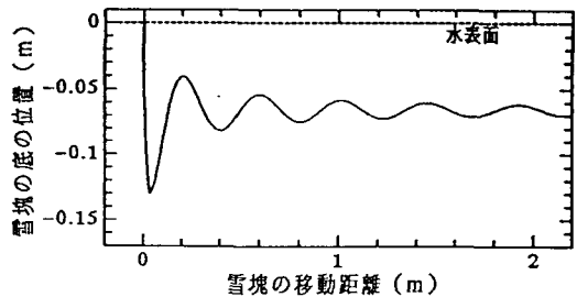
図-2 雪塊の上下変動特性
