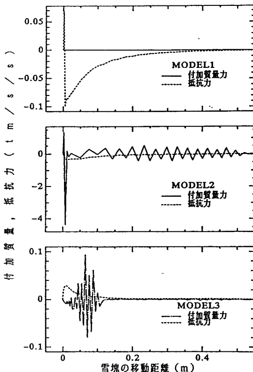
図-3 各モデルの付加質量力と抵抗力
