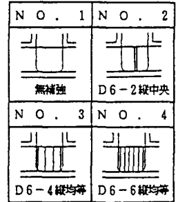
図-2 接合部帯鉄筋 の配置方法
