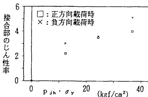
図-4 p_{jh} \cdot \sigma_y と接合部のじん性率
