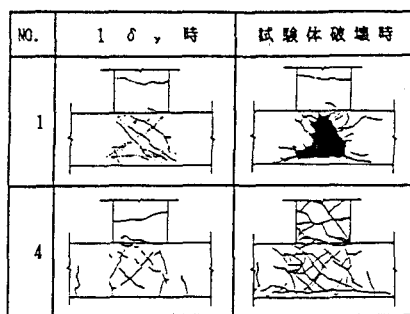
図-3 ひびわれ状況の例
