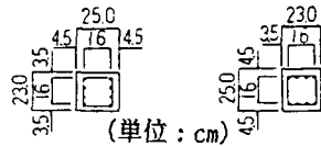
（単位：cm） 図-1 試験体の形状寸法
