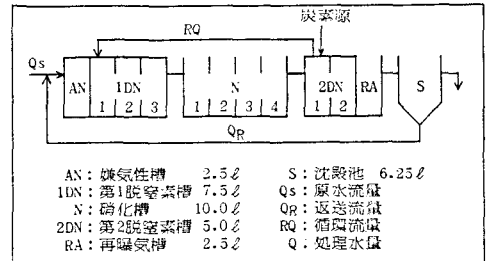
図-1 循環式硝化脱窒変法実験フロー
