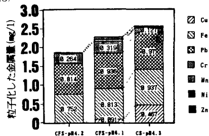
図-3 8時間における粒子化した金属量
