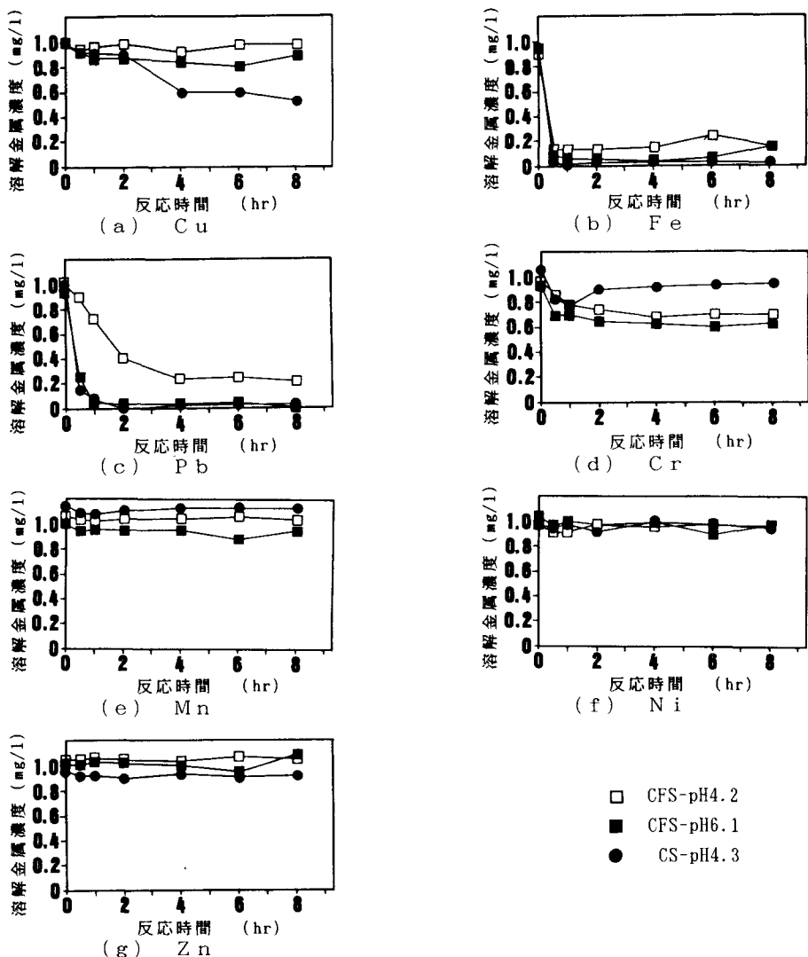
図-2 反応時間と溶解金属濃度 (a)～(g)
