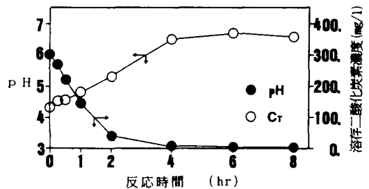
図-1 反応時間とpHおよびC T
