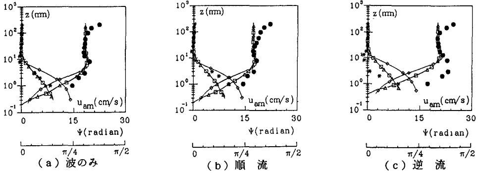
図-1 波動流速成分の振幅と位相のずれ
