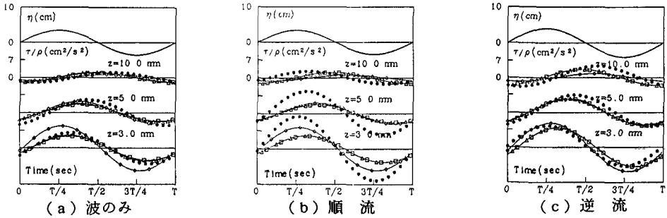
図-2 せん断応力
