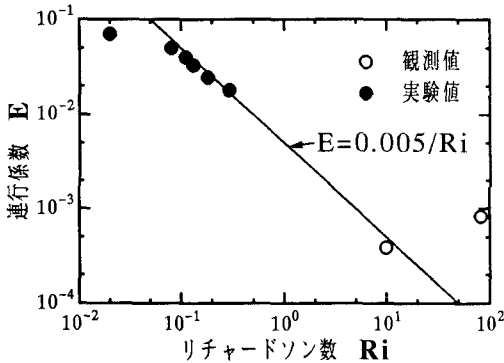
図-4 連行速度
