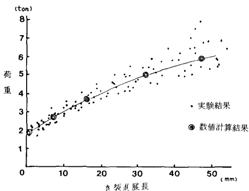
図-8 き裂進展長と荷重の対応
