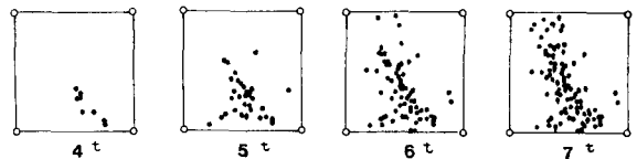
図-3 AE発生位置標定
