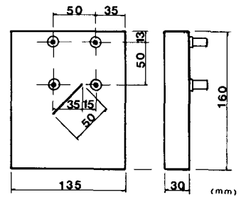
図-1 供試体
