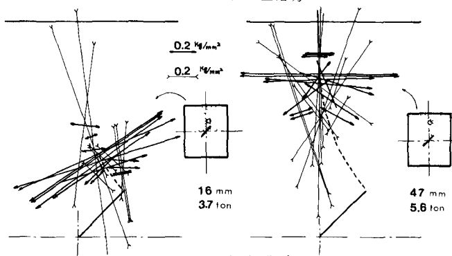
図-7 応力分布
