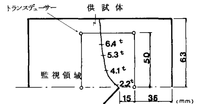
図-2 き裂進展図
