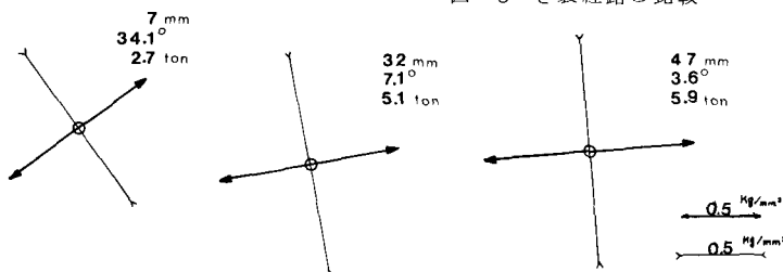
図-6 き裂先端近傍の主応力
