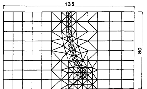
図-4 要素分割
