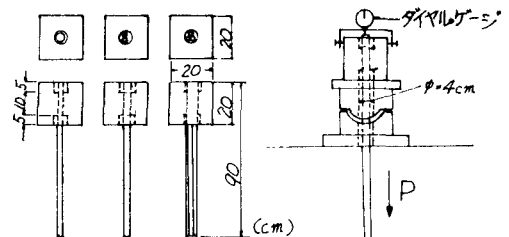
図-1 引抜き供試体
