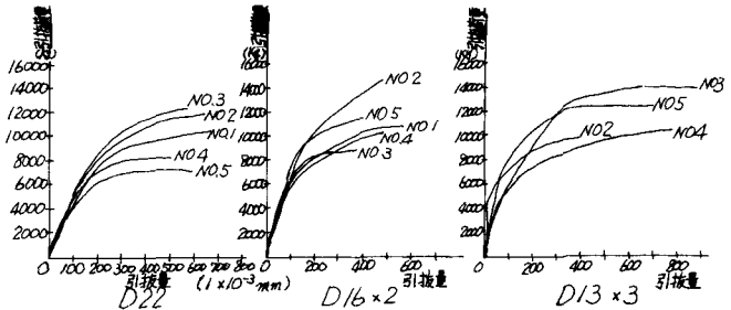
図-3 引抜き量-引抜き荷重曲線
