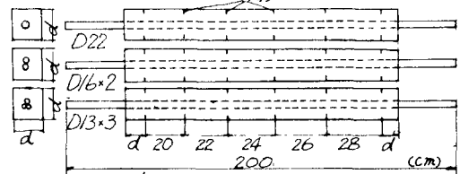
図-2 面引供試体
