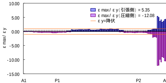
図 - 21 解析結果 (下弦材の最大ひずみ一覧) (CASE22)
