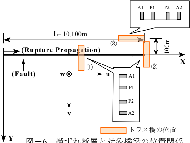
図－6 横ずれ断層と対象橋梁の位置関係
