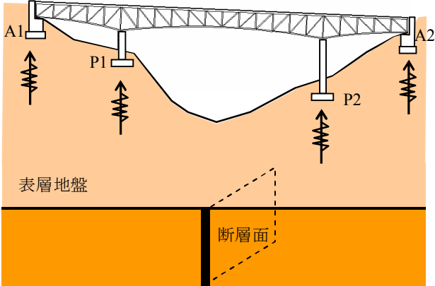
図－7 入力地震動の条件
