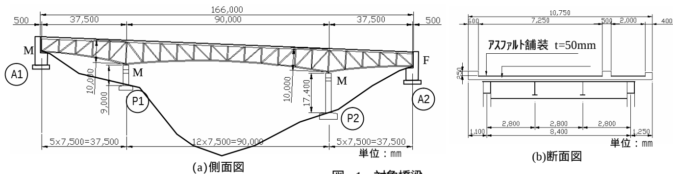
図 - 1 対象橋梁
