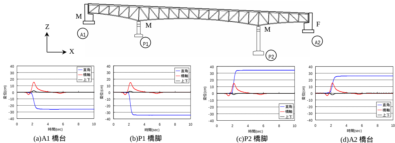
図 - 8 地震動変位波形 (CASE11)
