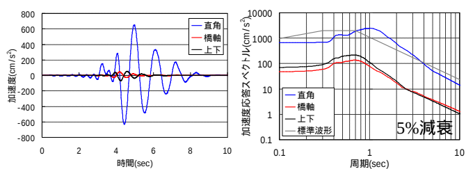
(a)地震加速度波形(P1) (b)加速度応答スペクトル(P1)
