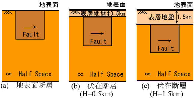
図－5 震源断層－地盤系モデル
