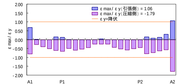
(b)垂直材の最大ひずみ一覧
