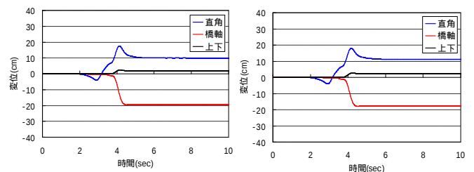
(a)P1 橋脚 (b)P2 橋脚
