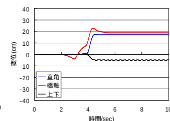
(b)P2 橋脚
