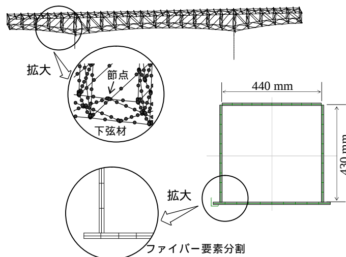
図 - 2 3 次元骨組モデル
