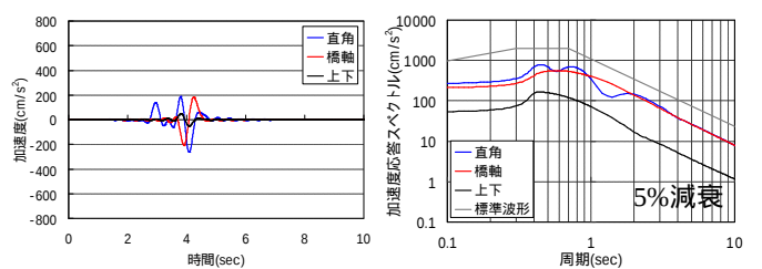
(a)地震加速度波形(P1) (b)加速度応答スペクトル(P1)
