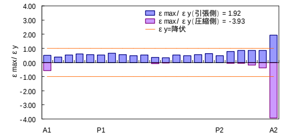
(c)斜材の最大ひずみ一覧
