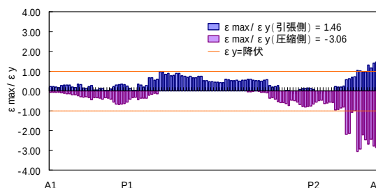
図 - 19 解析結果 (下弦材の最大ひずみ一覧) (CASE12)
