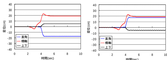
(a)P1 橋脚
