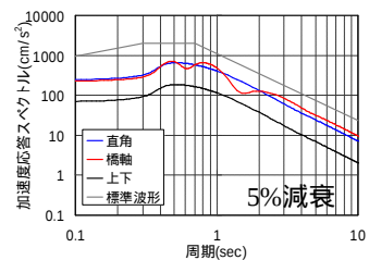
(b)加速度応答スペクトル(P1)
