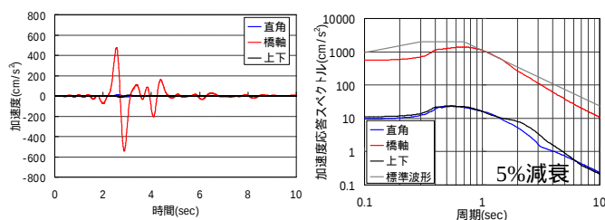
(a)地震加速度波形(P1)
