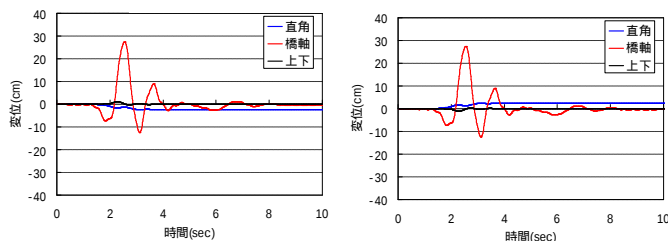
(a)P1 橋脚
