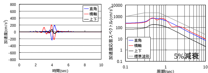
(a)地震加速度波形(P1)
