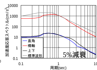
(b)加速度応答スペクトル(P1)
