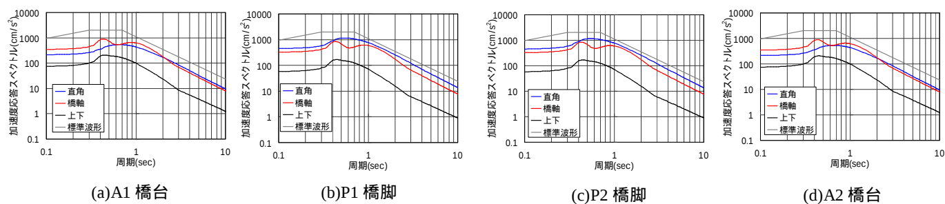
図 - 9 加速度応答スペクトル (5%減衰) (CASE11)
