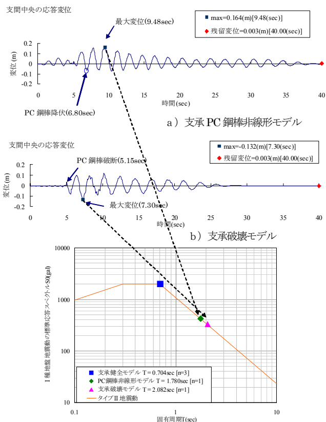
図-22 支承の破壊を考慮する場合の時刻歴応答変位と長周期化
