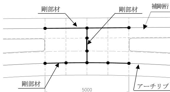
図－6 アーチクラウン部のモデル化
