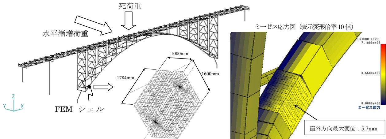
図-25 アーチリブに着目した面外変形量の算出
