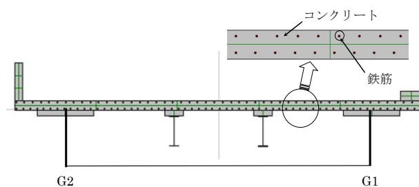
図－4 RC床版のモデル化
