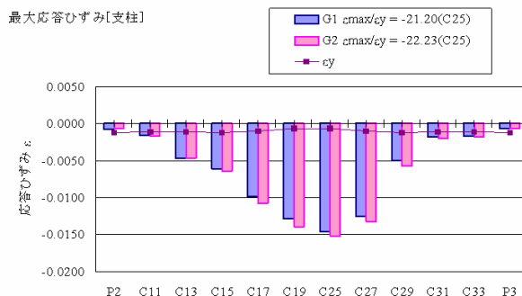
図-21 支承モデルの違いによるアーチ橋支柱部の最大ひずみ
