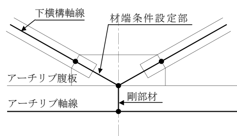
図－7 格点部のモデル化
