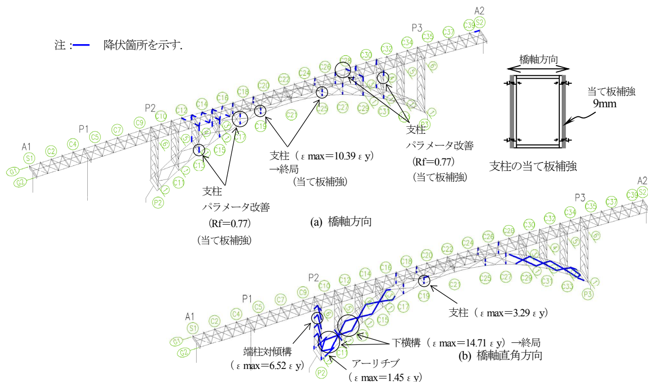
図-14 非線形時刻歴応答解析による塑性化の箇所
