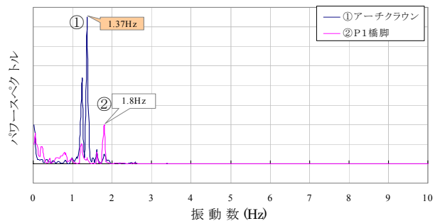
(a) 橋軸方向の卓越振動数
