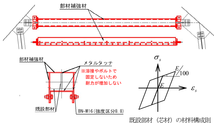
図-24 エネルギー吸収型の部材補強工法
