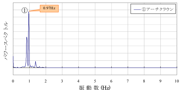
(b) 橋軸直角方向の卓越振動数
