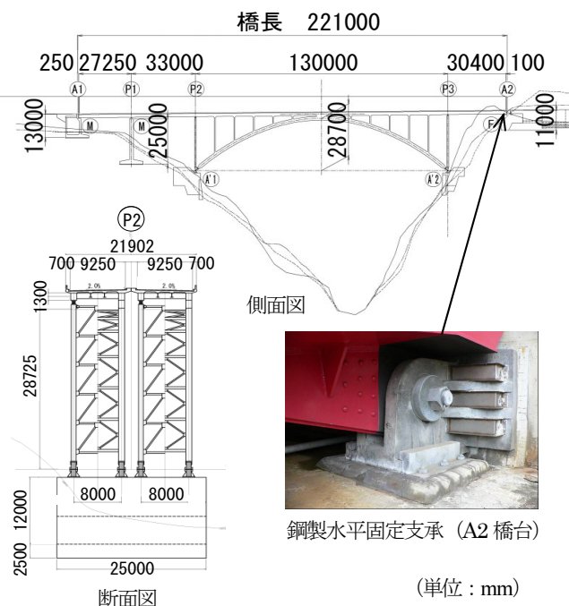
図-1 対象橋梁の一般図
