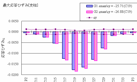
図-21 支承モデルの違いによるアーチ橋支柱部の最大ひずみ
