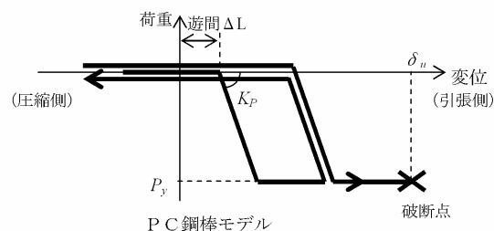
図-18 下横構の軸力-相対変位関係
