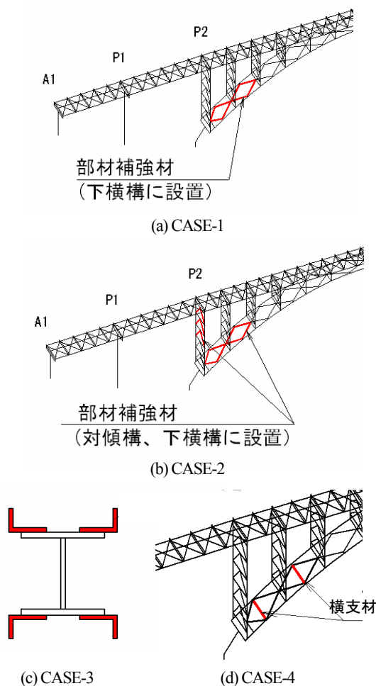
図-23 補強対策案
