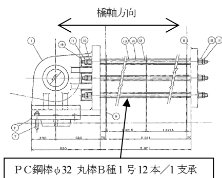
図-19 A2 橋台部の水平固定支承
