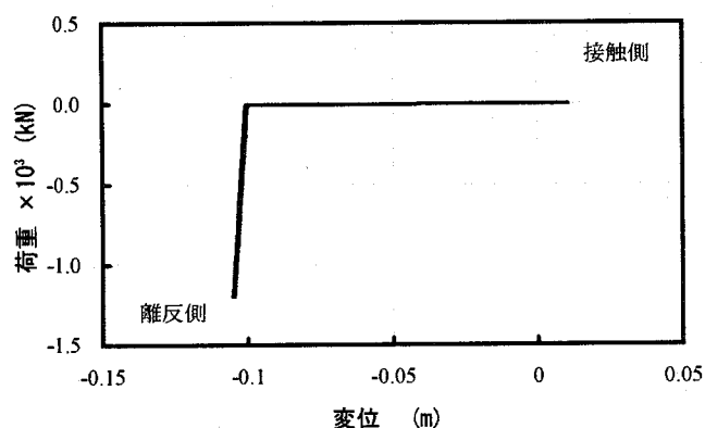
図-26 落橋防止装置の履歴図(Case4)
