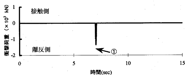
図-23 桁間の衝撃力の時刻歴応答(Case6)
