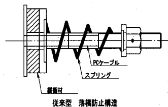
図-2 TE 型と従来型の構造
