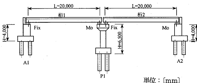
図-5 2径間単純桁橋の構造概要図
