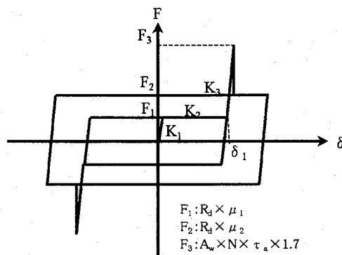
図-8 可動支承の復元力モデル
