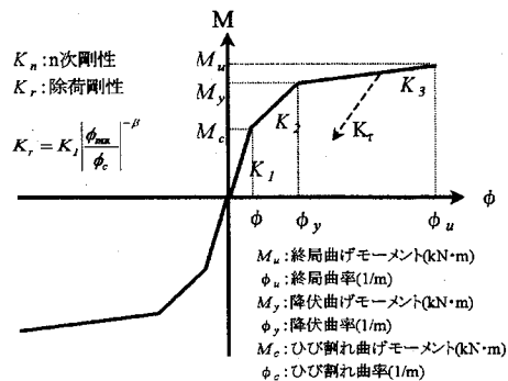
図-6 橋脚の復元力モデル
