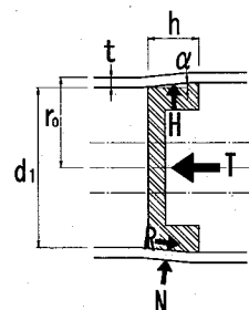
図-4 ウェッジプレートの摩擦抵抗抗図
