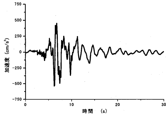
図-11 入力地震動（標準波形）
