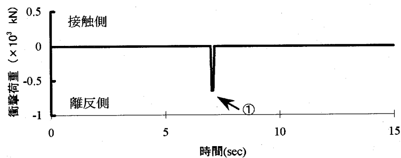
図-25 桁間の衝撃力の時刻歴応答(Case7)
