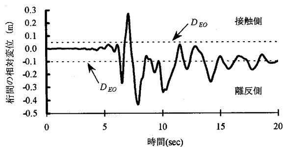
図-12 Case1 の時刻歴応答図
