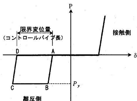
図-28 エネルギー吸収の概念図
