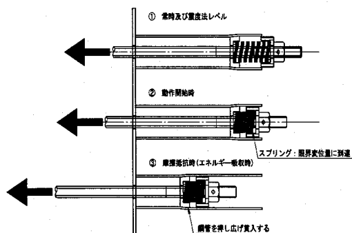
図-3 TE 型の荷重作用状況図
