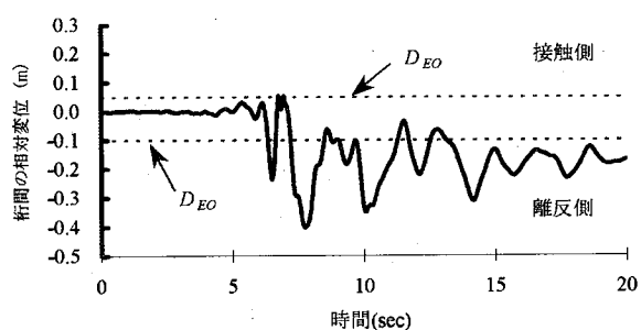
図-13 Case3 の時刻歴応答図
