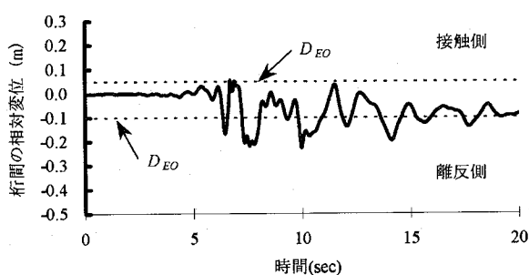
図-14 Case5 の時刻歴応答図
