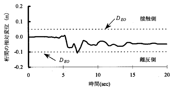
図-18 Case4 の時刻歴応答図
