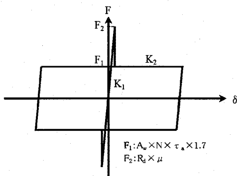
図-7 固定支承の復元力モデル
