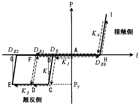
図-10 TE型の復元力モデル
