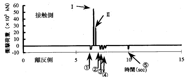
図-16 桁間の衝撃力の時刻歴応答(Case5)
