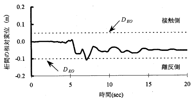
図-24 Case7 の時刻歴応答図
