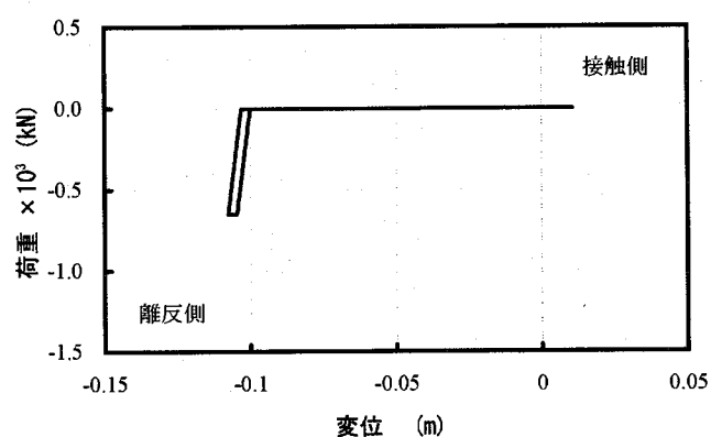
図-27 落橋防止装置の履歴図(Case7)
