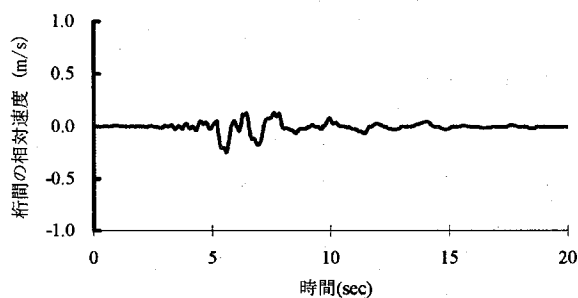
図-17 Case2 の時刻歴応答図
