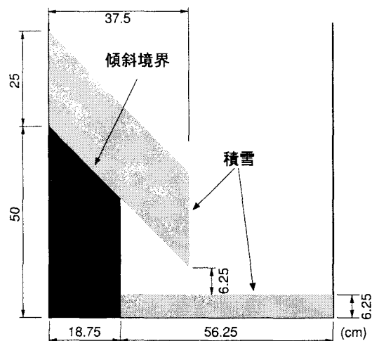
図-10 傾斜面上におかれた積雪の解析条件.
