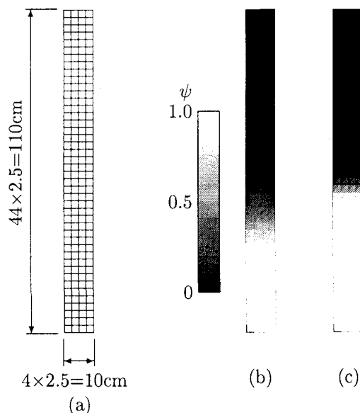
図-3 積雪柱の自重圧密解析. (a) 要素分割, (b) 移流計算に1次の風上差分を適用した場合, (c) 移流計算にCIP法を適用した場合 (いずれも t = 3.2 \times 10^5 \text{sec} における結果).
