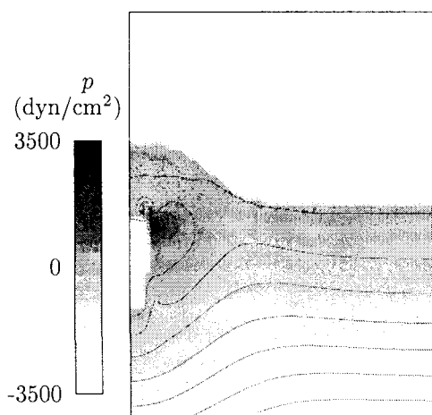
図-8 はりが埋設された積雪内の圧力分布 (3.7 日目).
