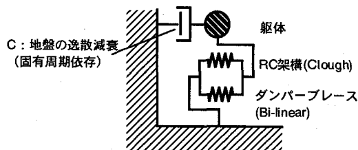
図-15 設計スペクトル解析モデル
