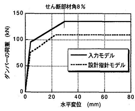
図-9 ダンパー・ブレースの入力モデル
