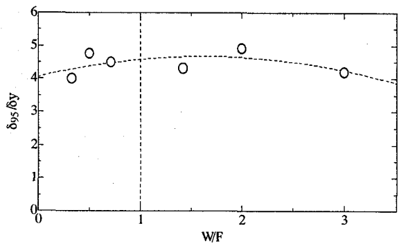
図-9 塑性率
