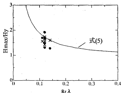
図-12 最大荷重推定
