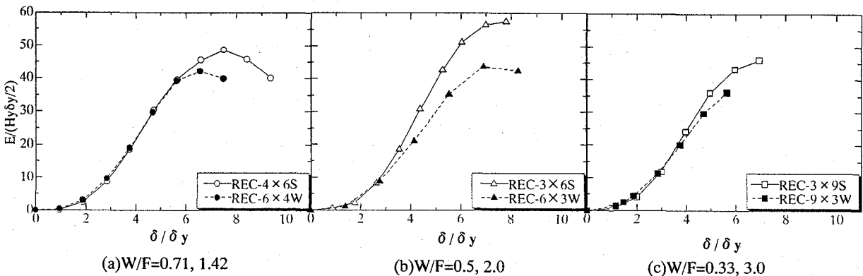
図-10 エネルギー吸収量
