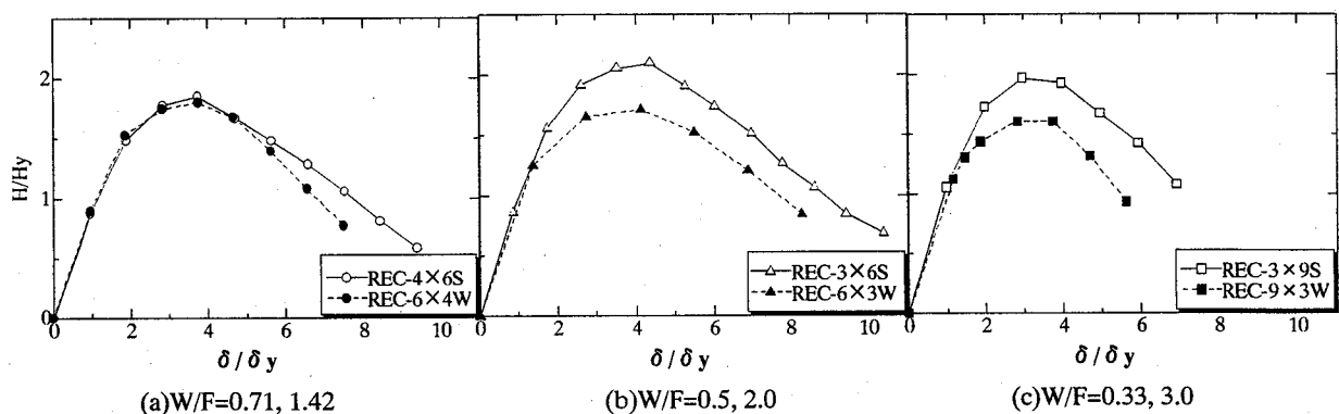
図-7 包絡線
