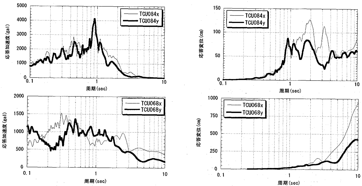
図-5 加速度及び変位応答スペクトル( h=2\% )
