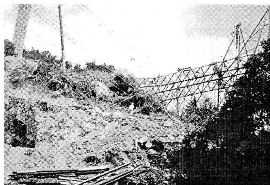
写真-1 倒壊した345kV超高压送電鉄塔 (中寮～峨眉間の#203)
