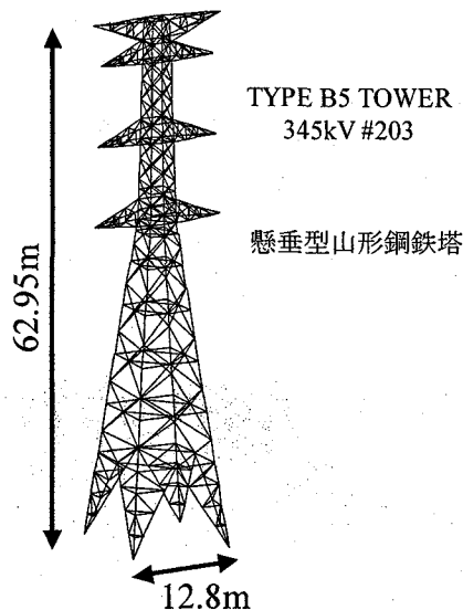
図-1 345kV鉄塔の構造概要
