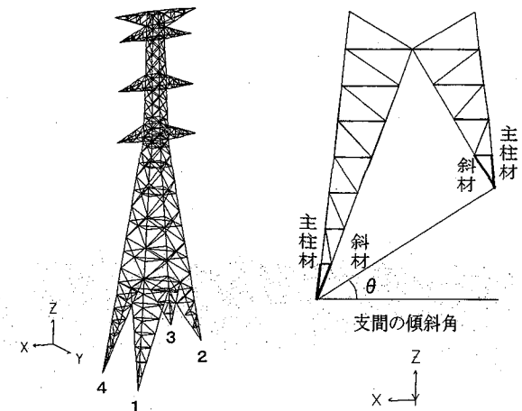
図-3 基部主柱材番号及び支間の傾斜角
