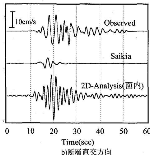
図-17 Sizukuishiにおける観測波と各手法により得られた解析波の比較
