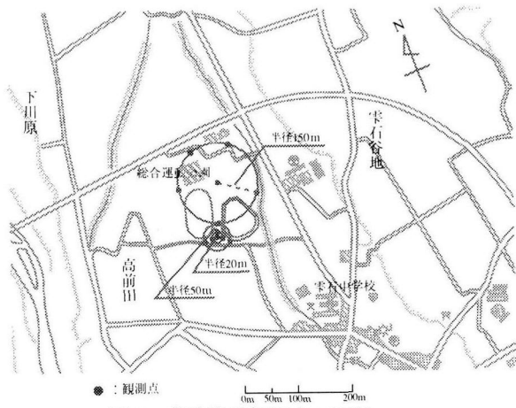
図-8 常時微動観測点の配置
