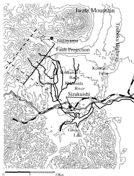
b)震源近傍における地震記録の観測位置
