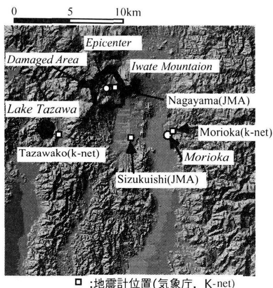
a)検討に用いた地震記録の全観測位置
