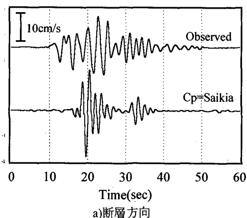
図-20 Saikia手法によるコントロール波に基づく疑似3次元解析による解析波と観測波の比較
