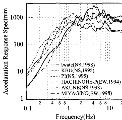
図-7 震度6弱を記録した既往の地震記録の加速度応答スペクトル( \eta=5\% )との比較
