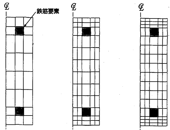
(a) 3 \times 8 分割 (b) 5 \times 12 分割 (c) 5 \times 16 分割 図-5 断面方向の要素分割ケース (A-Type 試験体)
