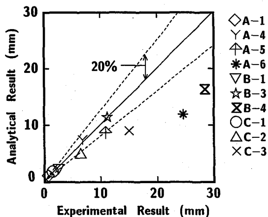
図-1 4 最大載荷点変位に関する比較
