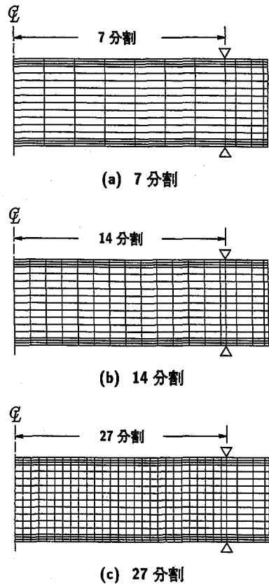
図-7 スパン方向の要素分割ケース (A-Type 試験体)
