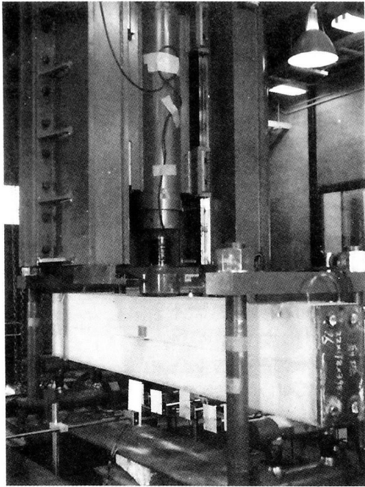
写真－１ 重錘落下衝撃実験の状況（A-Type 試験体）
