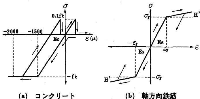
図-4 応力-歪特性
