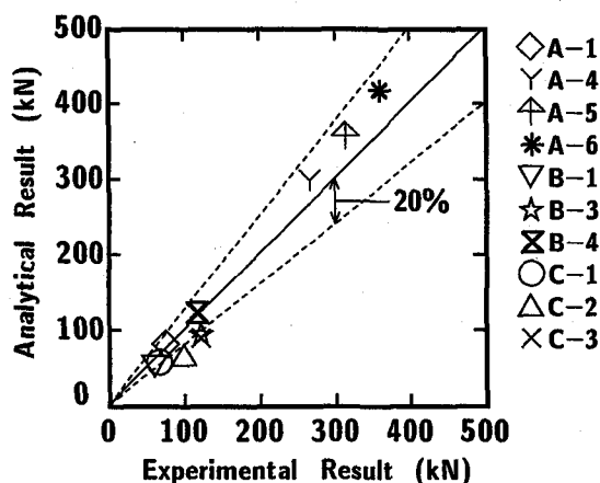
図-10 最大重錘衝撃力に関する比較
