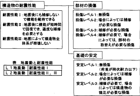
図- 24 耐震性能と損傷レベル
