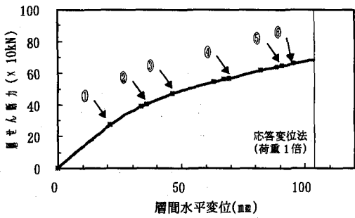
図- 22 荷重～変位関係（上沢駅）
