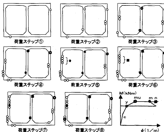
図- 14 損傷過程 (一般軌道部D 4)
