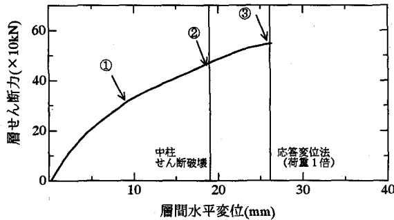
図- 5 荷重～変位関係(大開駅)
