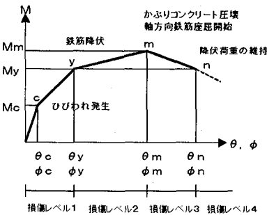
図- 25 地下構造物の耐震性能
