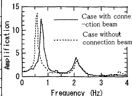
図-2 基盤に対する高架橋天端の周波数伝達関数 2)
