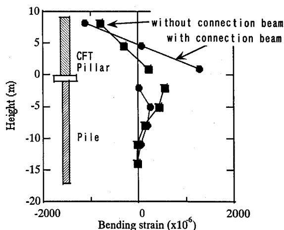
図-4 CFT柱・杭の曲げひずみ分布 2)
