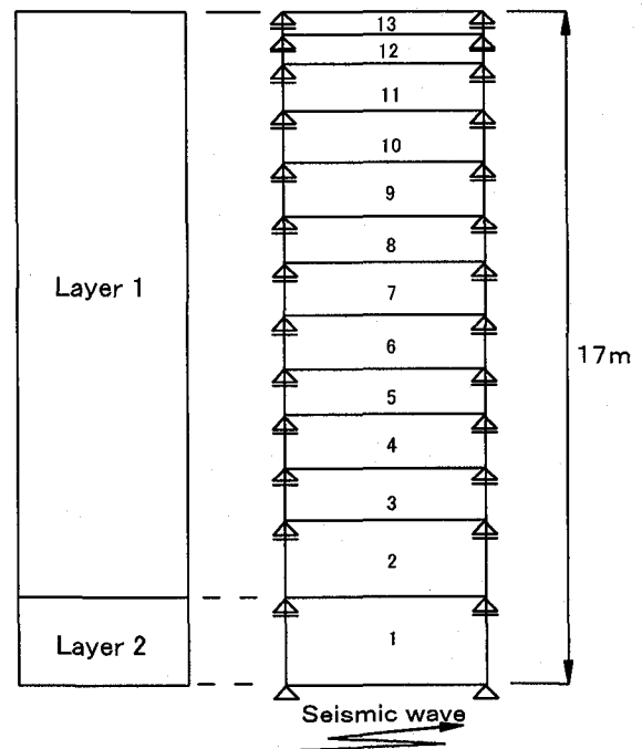
図-9 1次元非線形有限要素解析モデル
