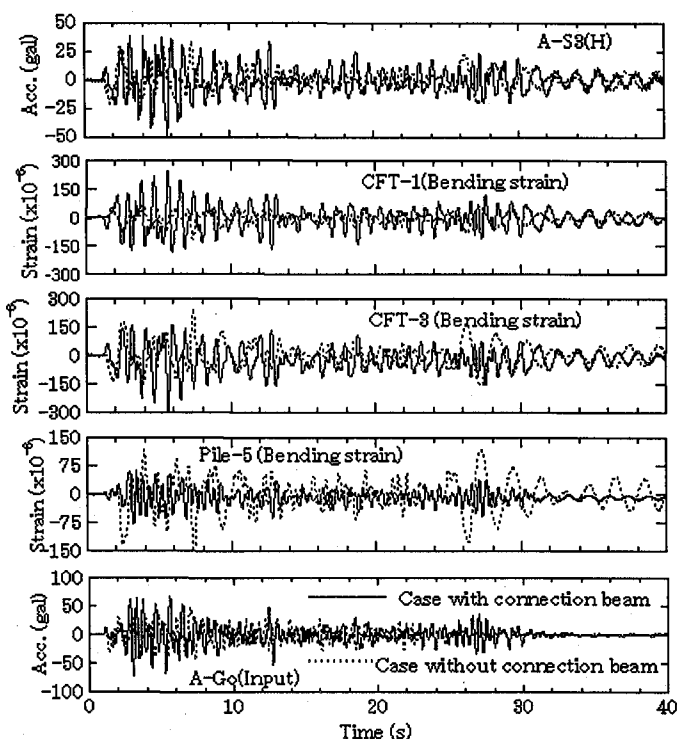
図-5 天端加速度・CFT柱・杭頭曲げひずみの応答
