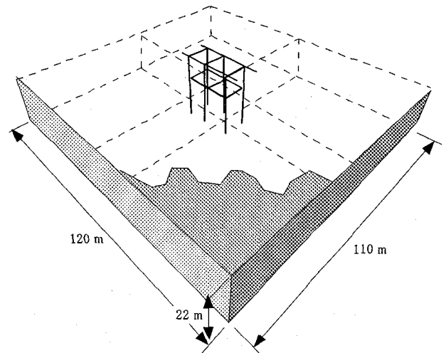
図-7 時刻歴応答解析用のFEM解析モデル
