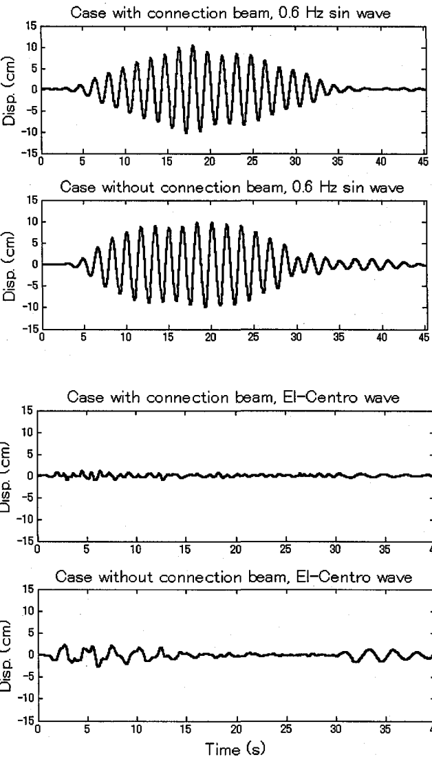
図-12 CFT柱頂部の水平変位の時刻歴（数値解析結果）
