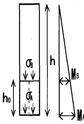
図-2 曲げモーメント分布と応力分布の関係
