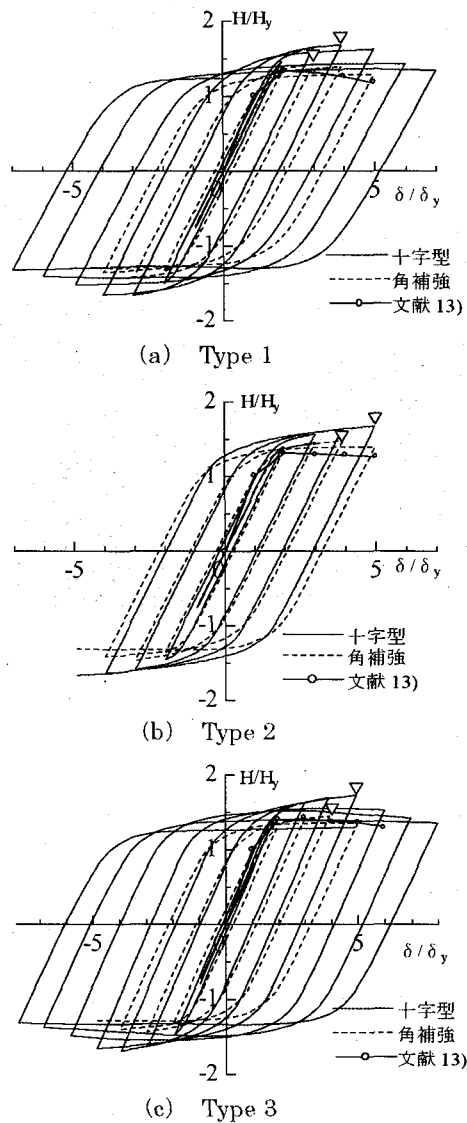
図-14 荷重-変位履歴曲線
