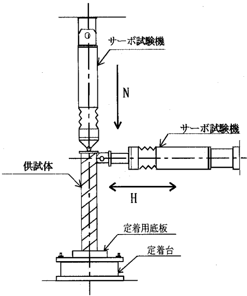
図-4 実験装置
