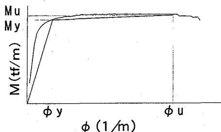
図-4 RC橋脚断面のM～φ関係
