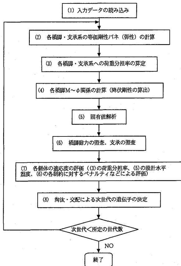
図-5 GAを用いた地震時保有水平耐力設計のフロー
