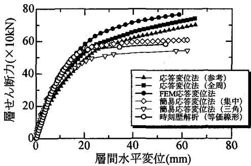
図-10 層せん断力～層間水平変位 (Case 2)
