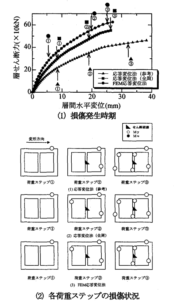
図-17 FEM 応答変位法および応答変位法の損傷状況
