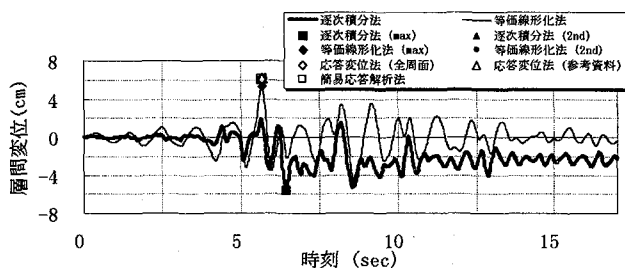
図-8 層間水平変位の時刻歴波形(Case 2)
