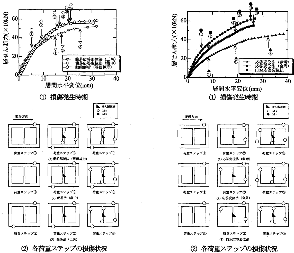
図-16 動的解析法および簡易応答変位法の損傷状況
