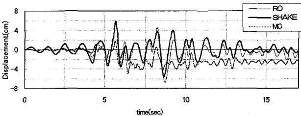
図-9 自然地盤での層間水平変位 (Case 2)
