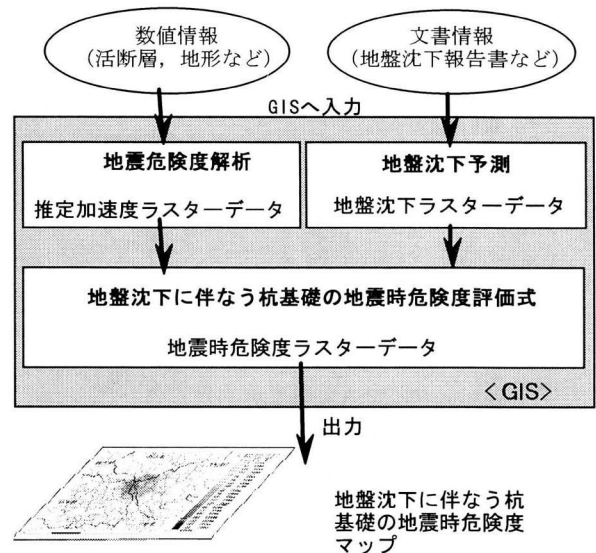
図-6 地盤沈下に伴う杭基礎の地震危険度マップ作成の流れ
