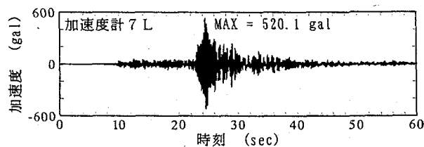
図-13 塔上部水平材の加速度波形（橋軸方向）
