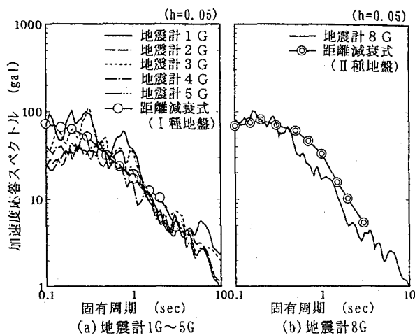
図-5 観測波の加速度応答スペクトル(鉛直方向)
