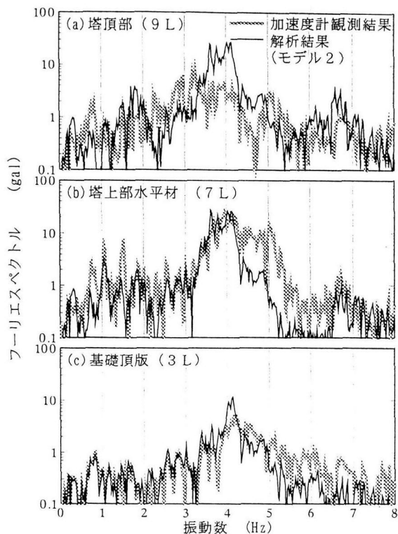
図-21 2P塔加速度波のフーリエスペクトル（橋軸方向）
