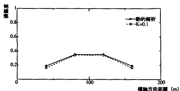
Kによる荷重比分布 (モデル1)
