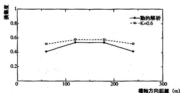
Kによる荷重比分布 (モデル2)
