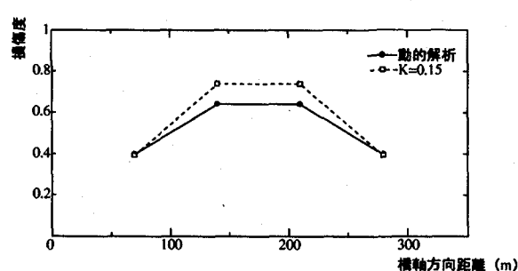
Kによる荷重比分布 (モデル3)
