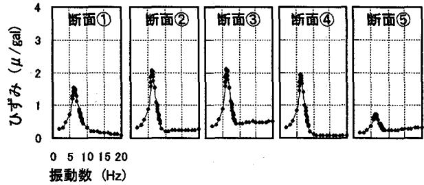
図-11 ひずみの共振曲線 (実験 J2, 二次覆工)
