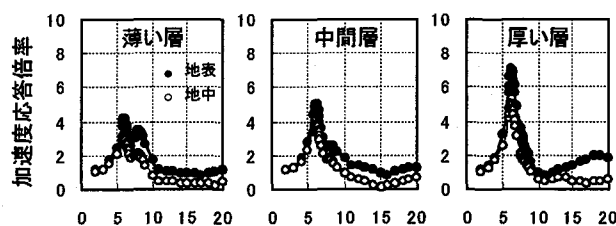
図-8 加速度の共振曲線 (実験 J2)
