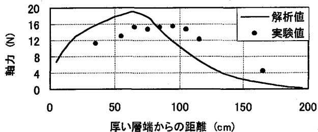
図-13 一次覆工の軸力 (実験 J1)
