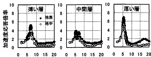
図-6 加速度の共振曲線 (実験 J)
