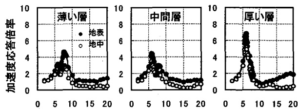
図-7 加速度の共振曲線 (実験 J1)
