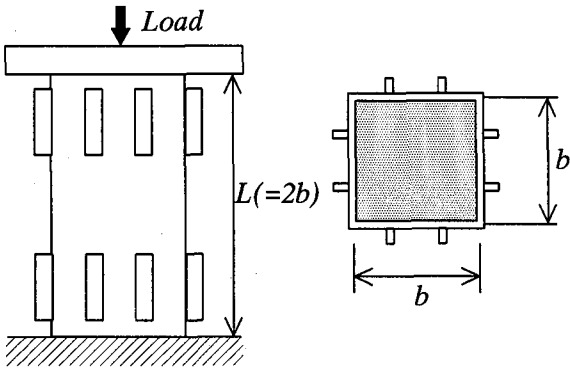
(a) 実験の概要 (b) 供試体断面図 図-8 実験の概要と解析モデル（解析例Ⅰ）
