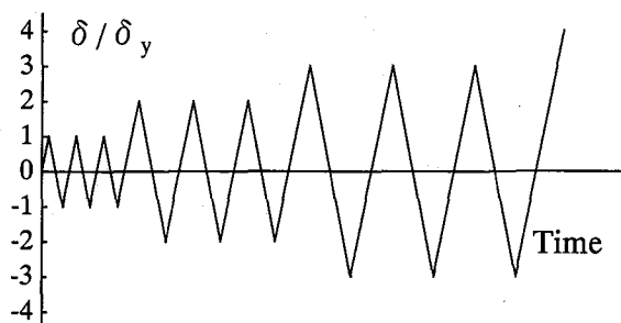
図-11 繰返し水平力の載荷方法（解析例Ⅱ）
