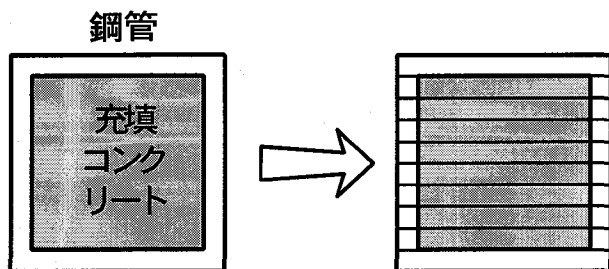
図-1 断面分割法
