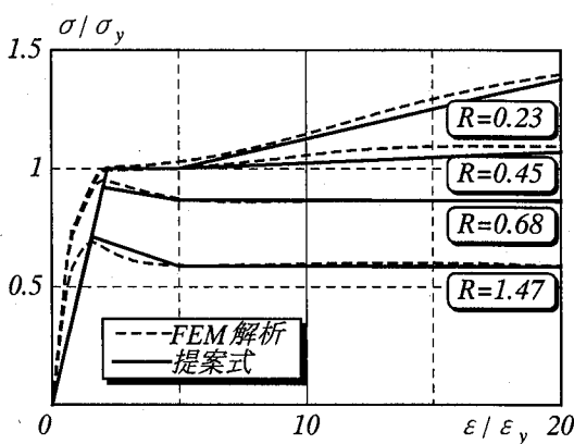
図-5 FEM 解析の結果と提案式との比較(SM490)
