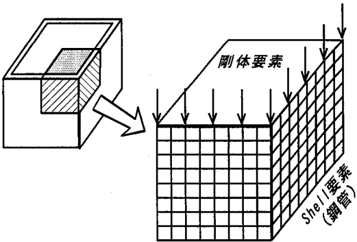
図-4 鋼管の FEM 解析モデル
