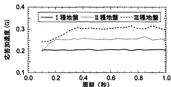
図-5 L 1 標準地震波の応答スペクトル
