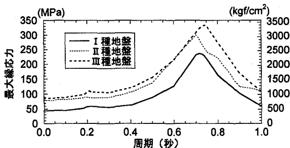
図-12 L1地震波に対する付属構造物の基部応力
