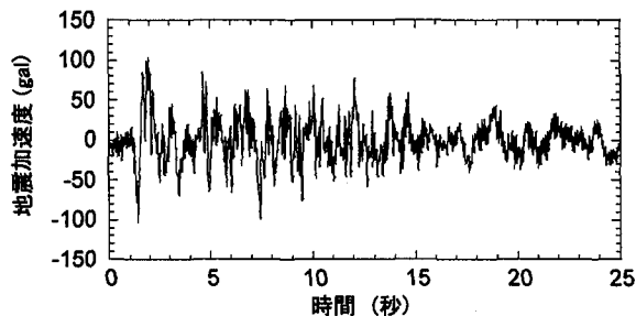
(a) I 種地盤用波形
