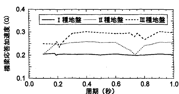
図-13 L1地震波に対する橋梁の加速度応答
