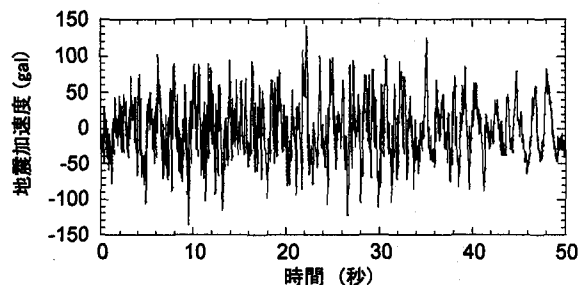
(c) III 種地盤用波形
