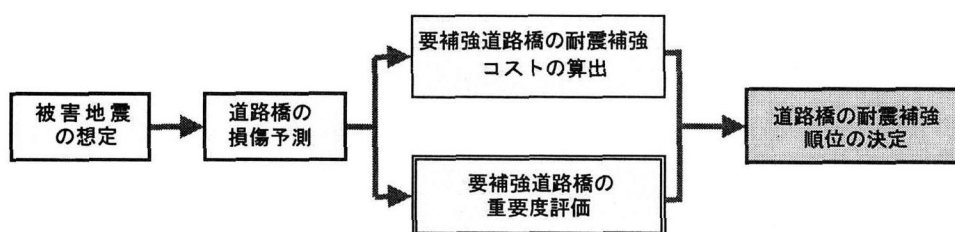
図-1 既設道路橋の耐震補強順位決定の流れ
