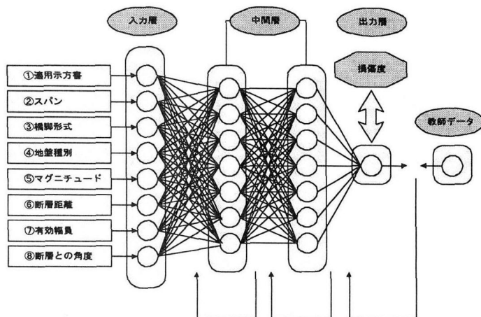
図－3 ネットワークモデル
