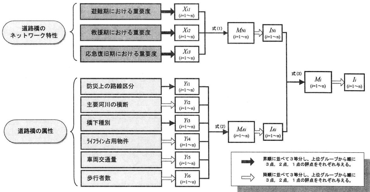
図－８ 道路橋の重要度 ( I_i, i=1\sim n ) の算定方法
