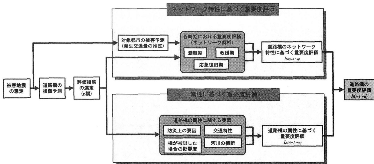
図－2 道路橋の地震防災上の重要度評価手順
