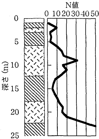
図3 地盤条件
