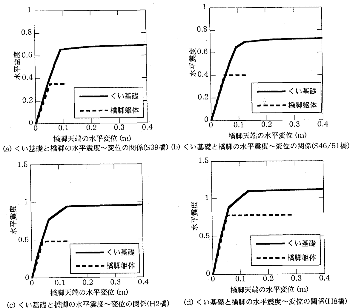
図8 くい基礎と橋脚の水平震度～水平変位の関係
