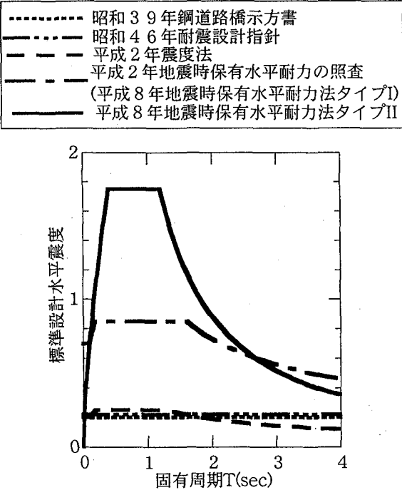
図1 解析対象とした基準に規定される設計水平震度 (II種地盤の場合)
