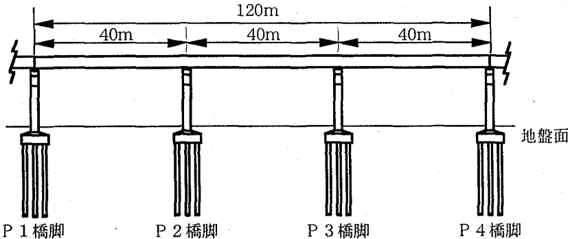
図2 解析の対象とする3径間連続鋼鈑桁橋
