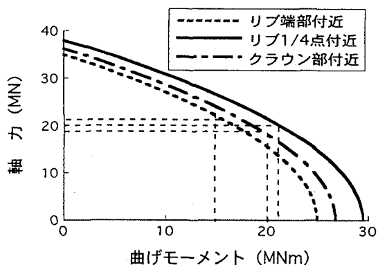
図-7 アーチリブのN-M関係曲線
