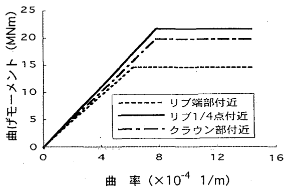
図-8 アーチリブの完全弾塑性バイリニアモデル
