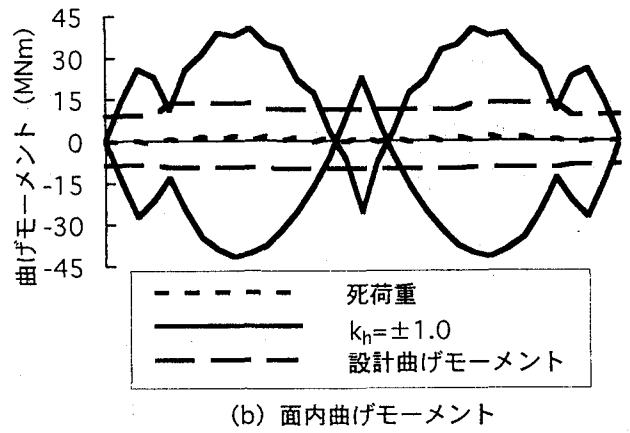
図-5 水平震度±1.0に相当する水平力を静的に作用させた場合の断面力
