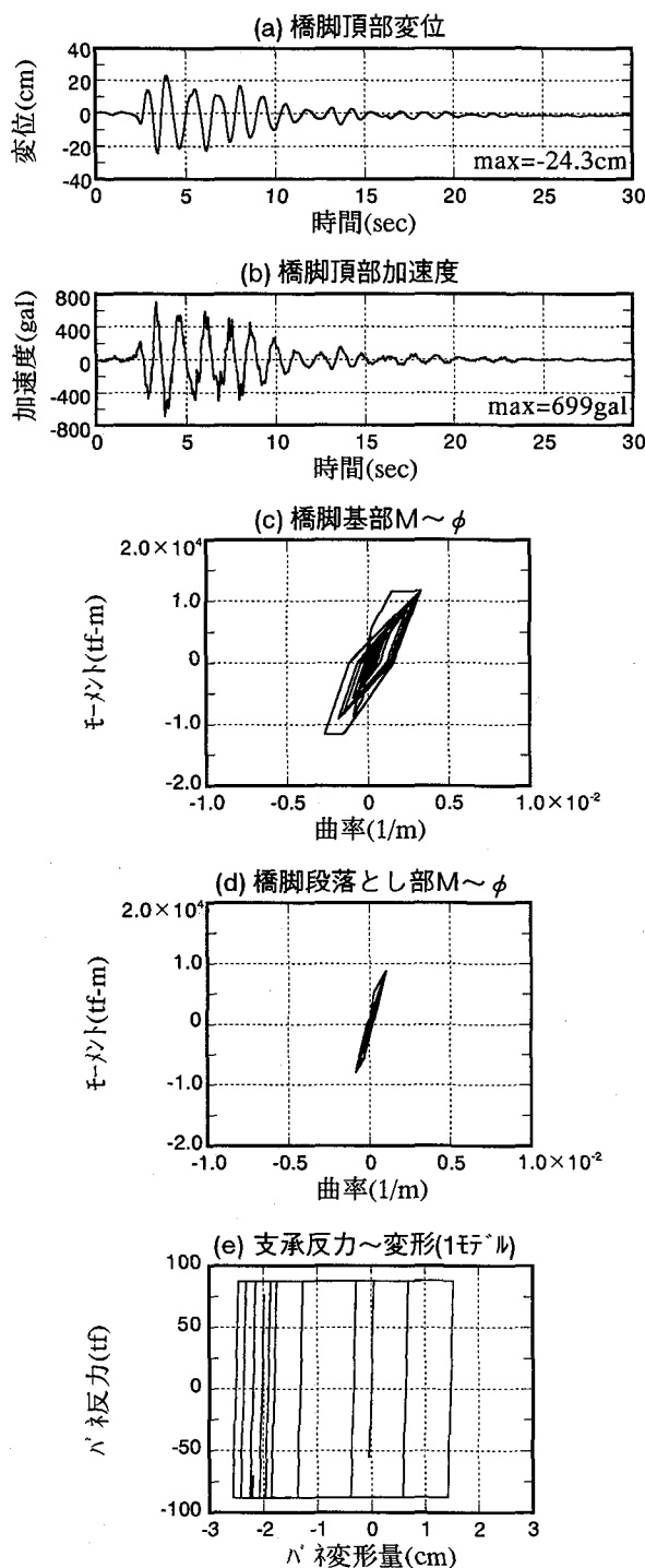
図—17 地震応答解析結果 ケース5：支承破断の影響
