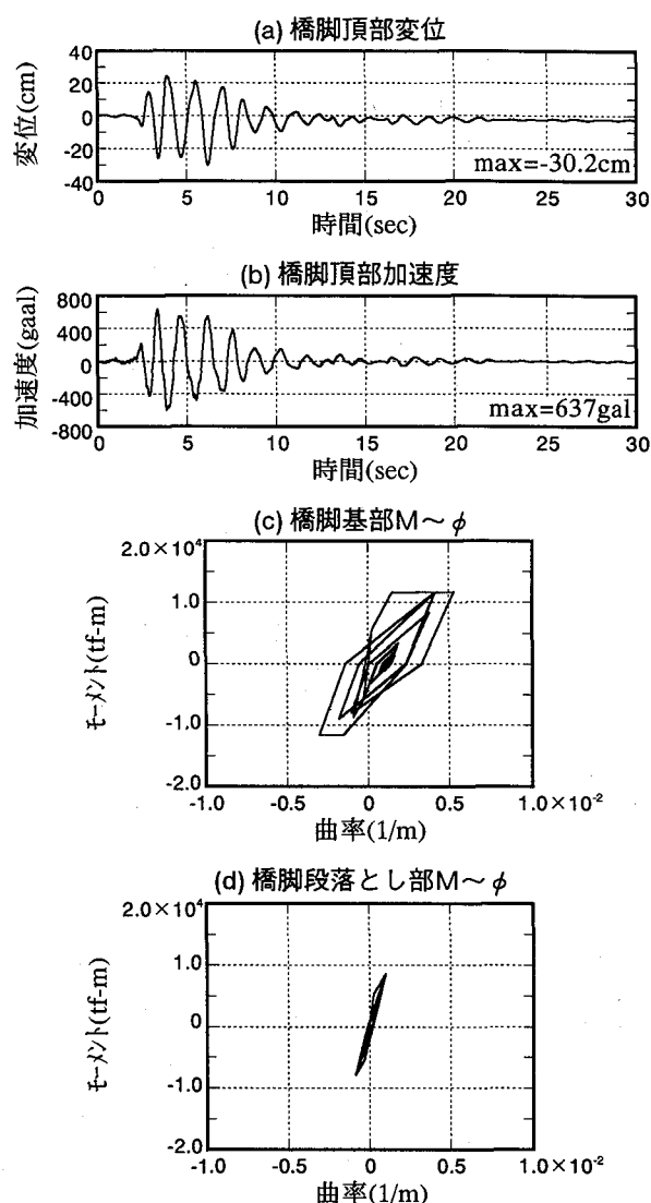
図一14 地震応答解析結果 ケース2：杭頭ひび割れの影響
