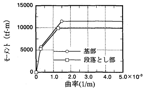
図一九 橋脚断面のモーメント～曲率 ( M \sim \phi ) 関係
