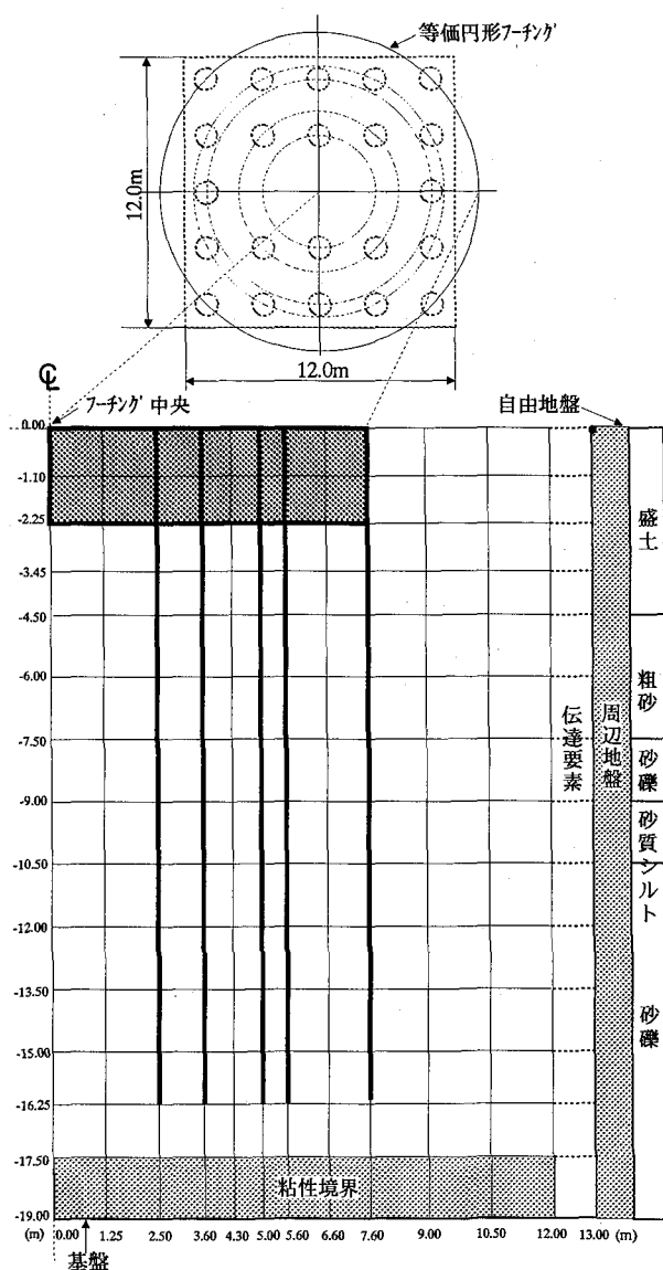
図一5 等価円形基礎と基礎～地盤系軸対象FEMモデル
