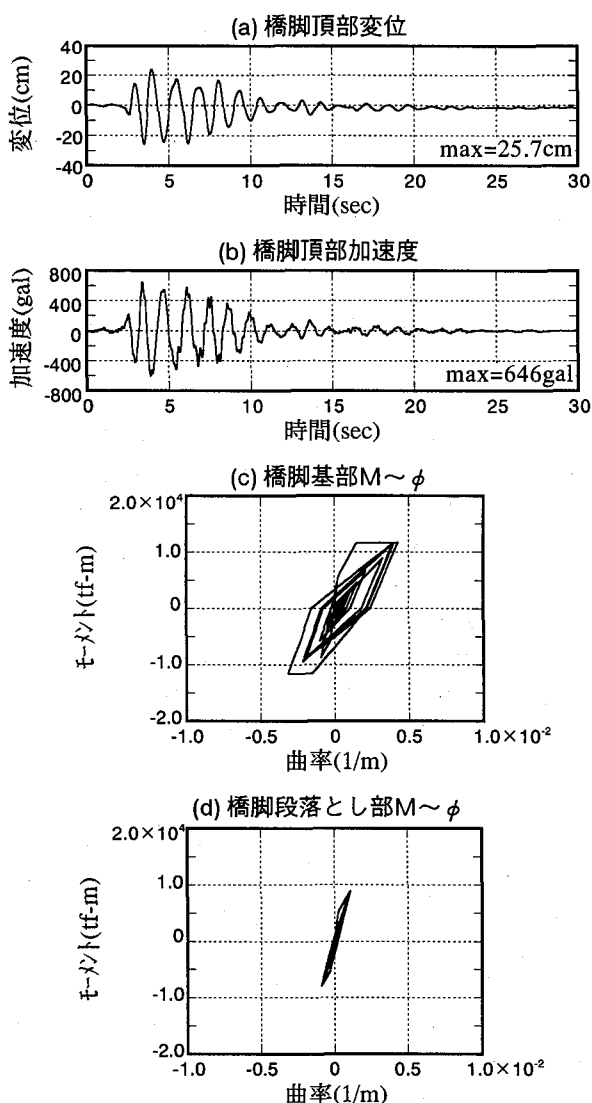
図一13 地震応答解析結果 ケース1：基本モデル
