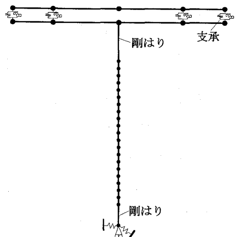
図一十一 動的解析用質点系モデル
