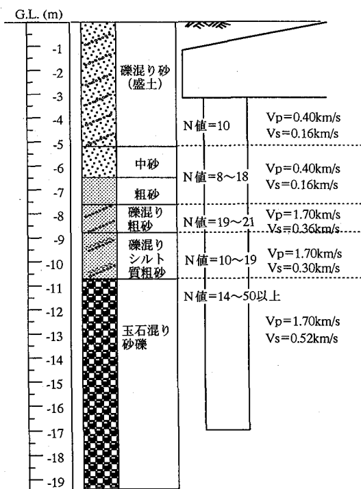
図—2 地盤ボーリング柱状図
