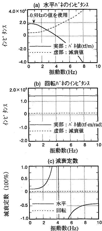
図一八 地盤の復素剛性
