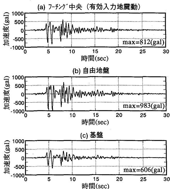
図一6 有効入力地震動
