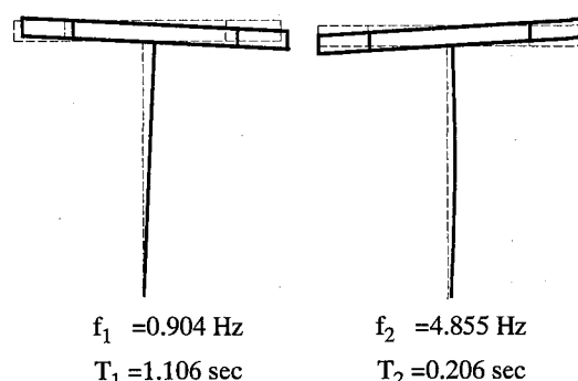
図—12 一次と二次モード型
