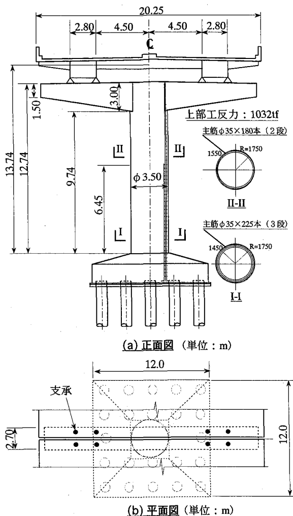
図—1 解析対象のT型単柱RC橋脚
