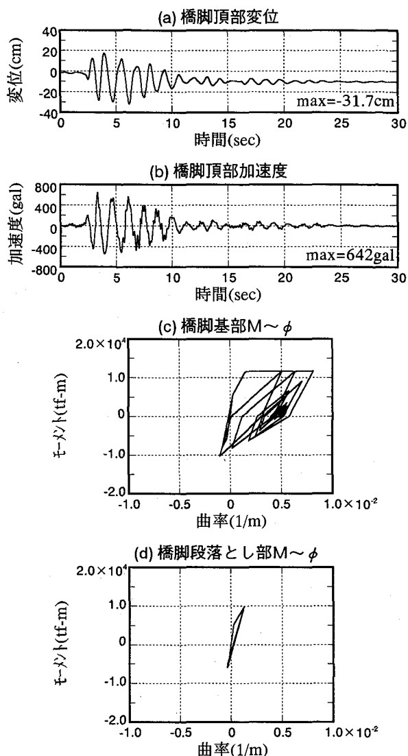
図—18 地震応答解析結果 ケース6：桁偏心（山側）の影響
