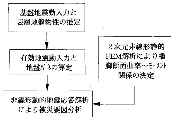
図—3 解析フローチャート
