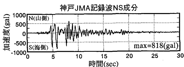
図一4 入力波：神戸海洋気象台NS成分
