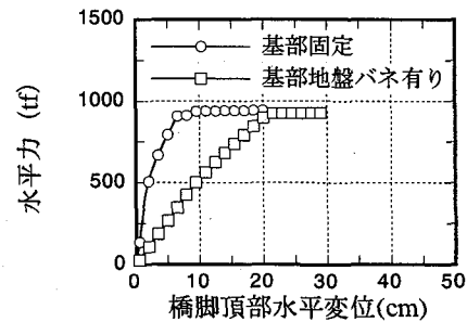
図一十 橋脚頂部水平力～変位 ( P \sim \Delta ) 関係
