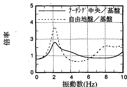
図一7 基礎、地盤の伝達関数
