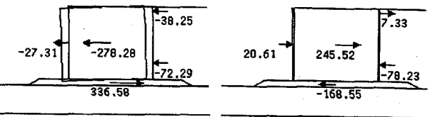
c) 400Gal 時 (変位 20 倍表示)
