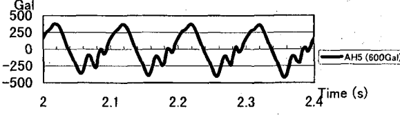
図 16 応答加速度（転換時、戻り波形）
