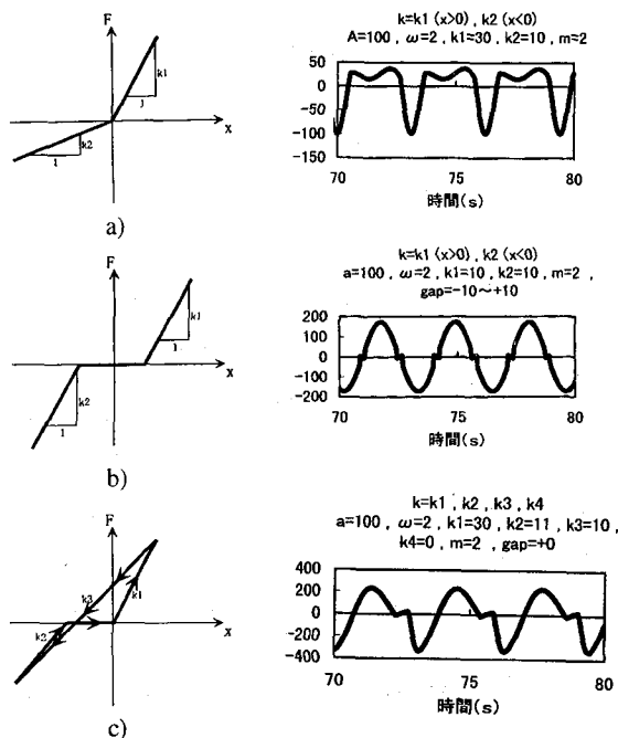
図 17 非線形バネとその時の応答加速度
