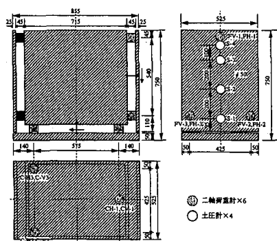
図1 模型の緒元
