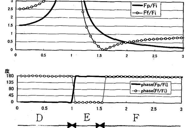
図 22 背面土圧と底面摩擦力の特性
