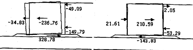
e) 800Gal 時 (変位 20 倍表示)
