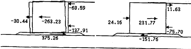
d) 600Gal 時 (変位 20 倍表示)
