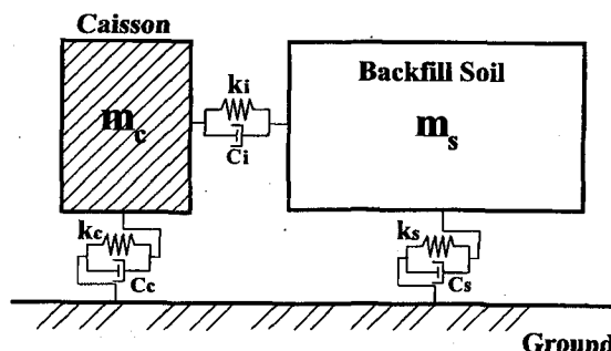
図 21 2 質点モデル
