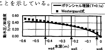
図 18 ケーソン水平運動による動水圧
