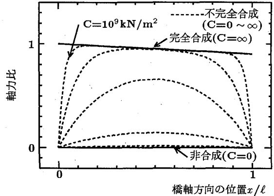
図-9 橋軸方向の軸力分布
