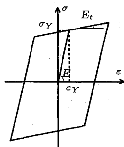
図-2-a 鋼材
