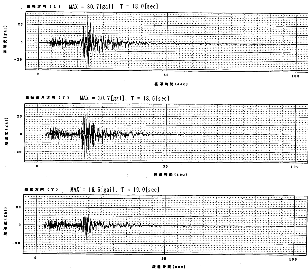
図-6 入力地震波
