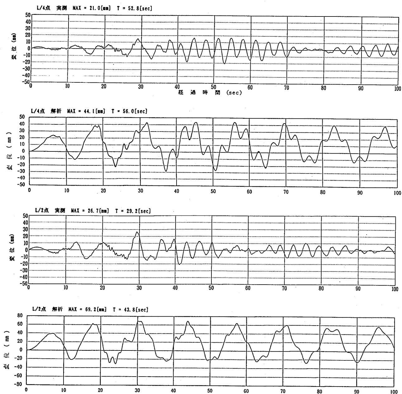
図-9 補剛桁の橋軸直角方向変位
