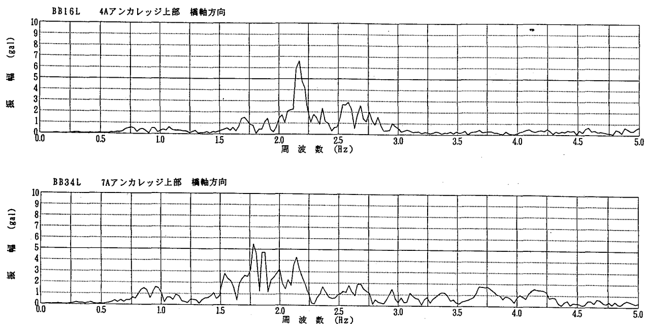
図-5 アンカレッジにおける相対加速度応答のフーリエスペクトル
