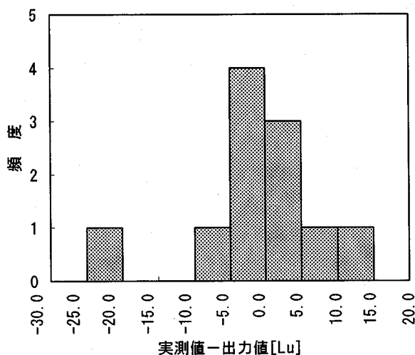
図-8 検証データの誤差分布
