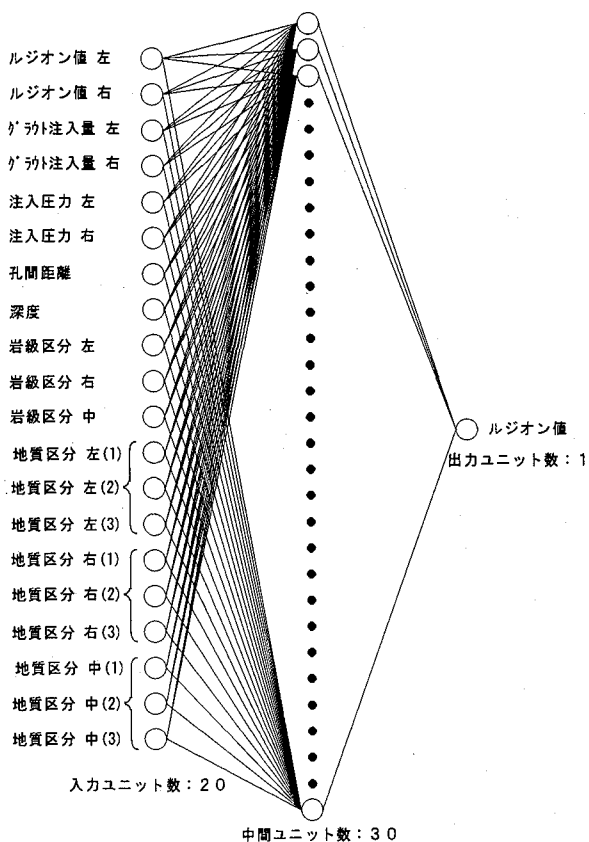
図-3 ニューラルネットワークのシステム構造
