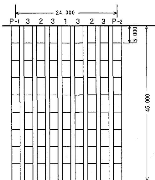
図-1 グ라우チング孔の配置
