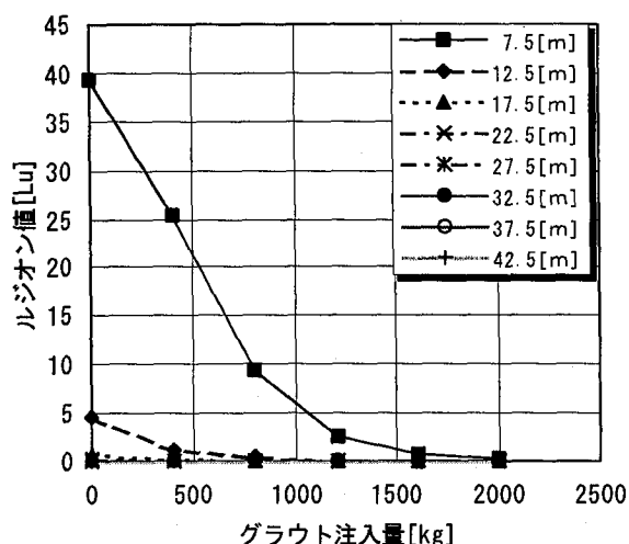
図-9 ルジオン値とグラウト注入量の関係
