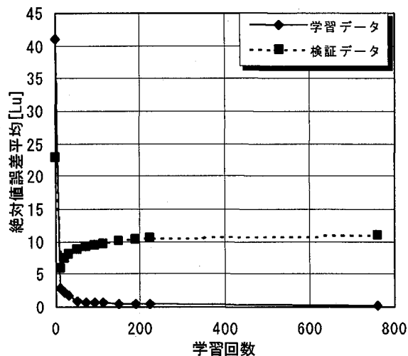
図-4 絶対誤差平均と学習回数
