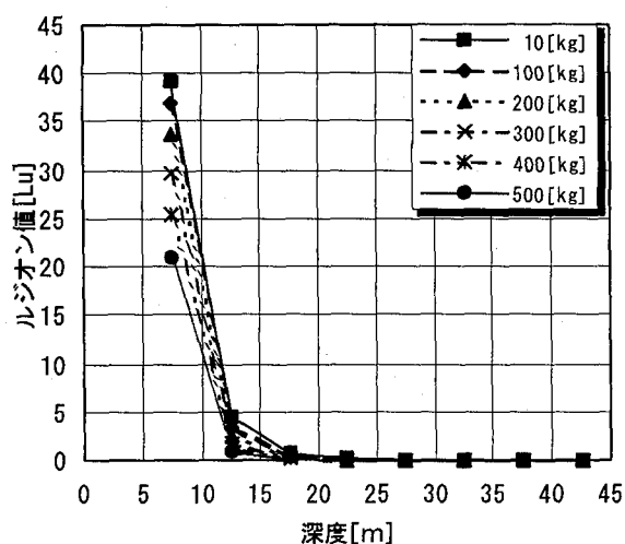
図-10 ルジオン値と深度の関係
