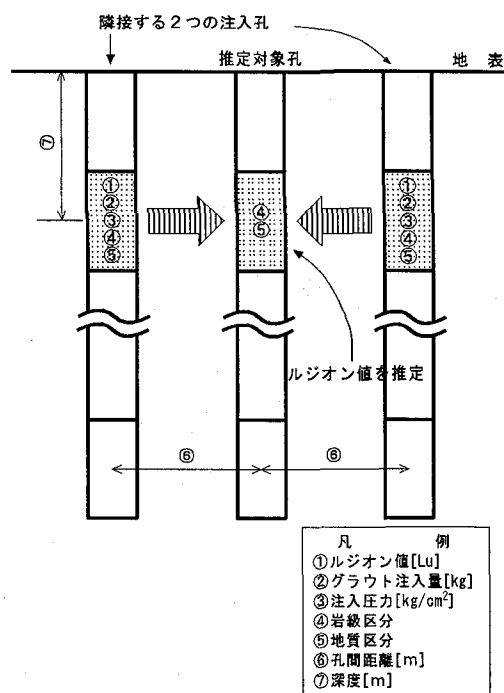
図-2 入出力項目の関係
