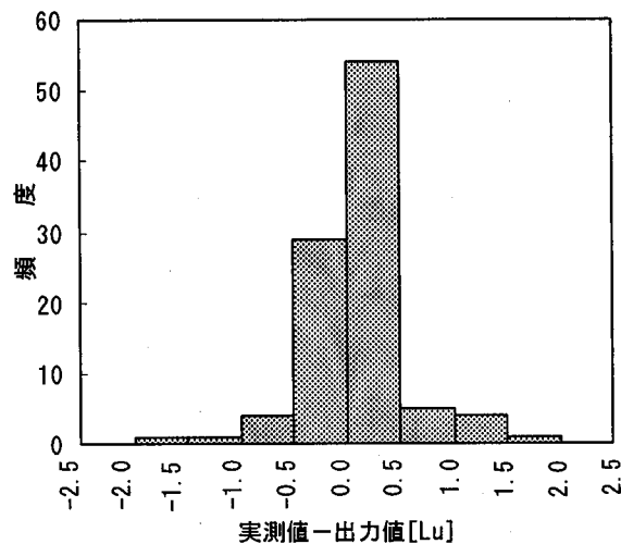
図-7 学習データの誤差分布
