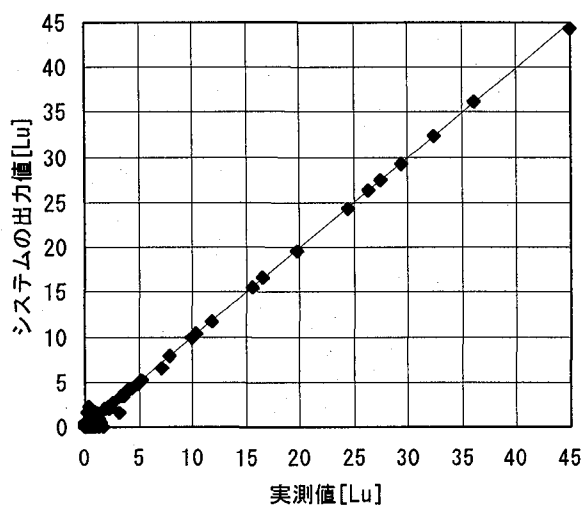
図-5 システムの出力値と実測値 (学習データ)
