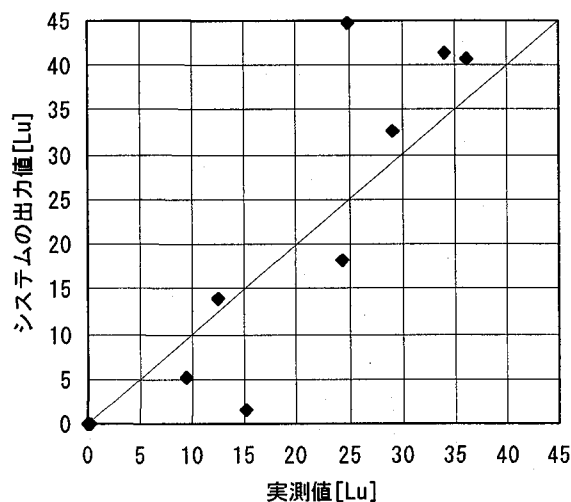
図-6 システムの出力値と実測値 (検証データ)
