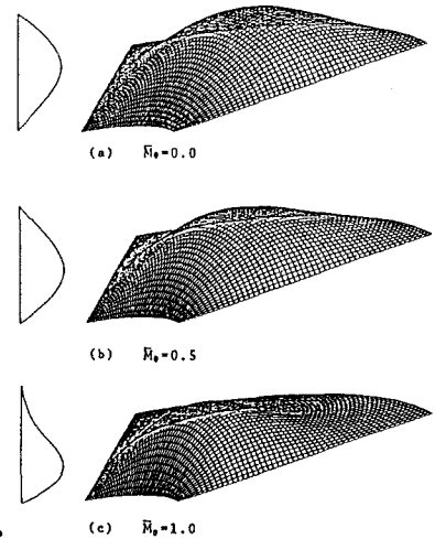
図-3 静的曲げモーメントの変化に伴う固有振動形の変化(case I)
