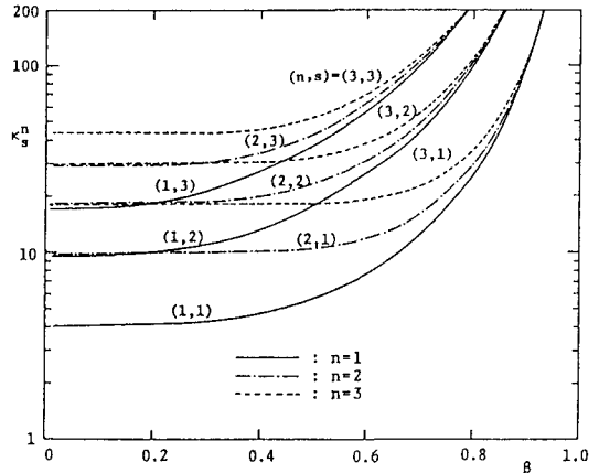
図-5 内外径比の変化に伴う固有振動数の変化(case I, \alpha=60^\circ )
