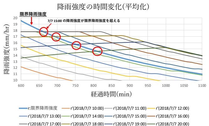
図-6 限界降雨強度と平均化した降雨データの比較
