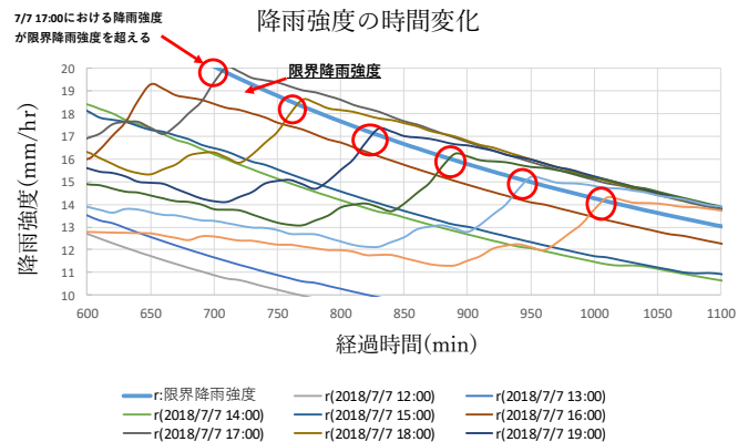
図-5 限界降雨強度と降雨データの比較
