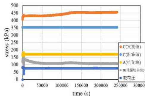
図5 40~80kPa 載荷時の各地点の応力
