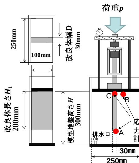
図3 実験装置概略図
