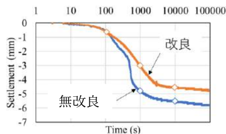
図4 40~80kPa 載荷時の地表面沈下量
