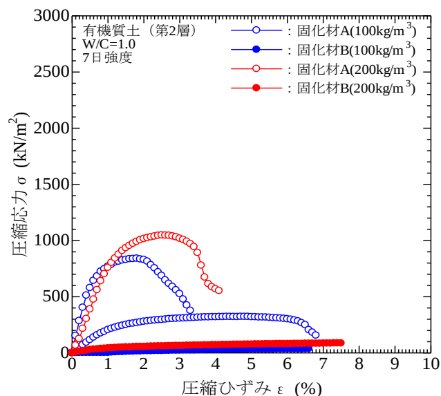
図-2 応力-ひずみ曲線
