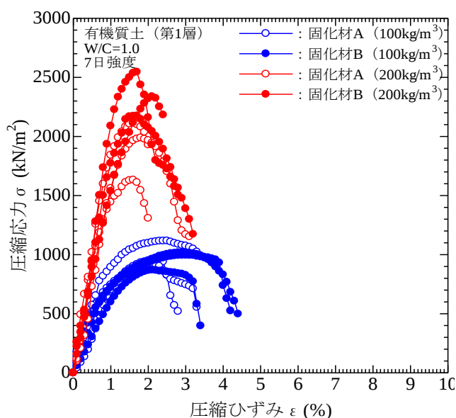
図-1 応力-ひずみ曲線
