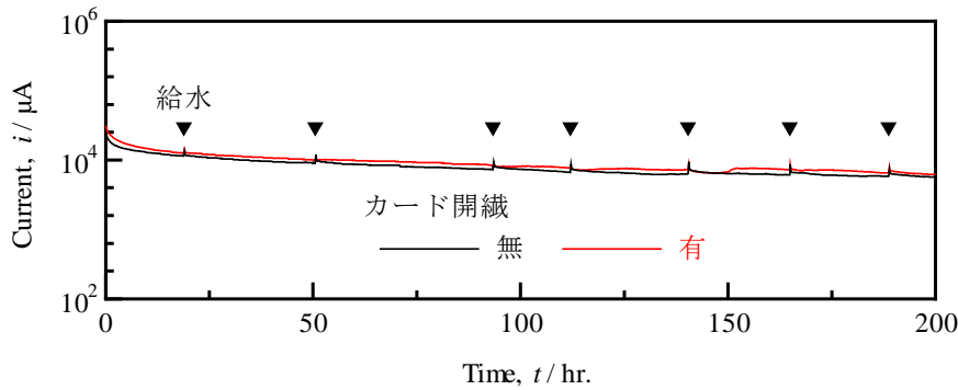
図-3 防食電流の経時変化
