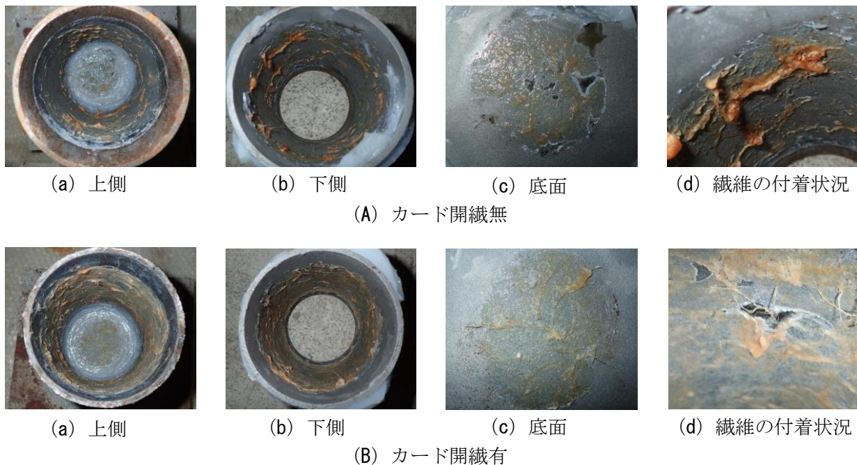
図-4 試験体の防食状況と繊維の付着状況（試験開始から 540 時間後）
