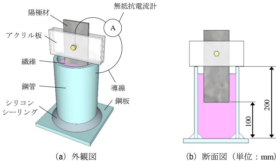
図-1 試験体の概略図
