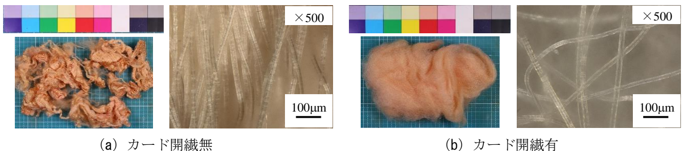
図-2 繊維（架橋型アクリレート繊維）
