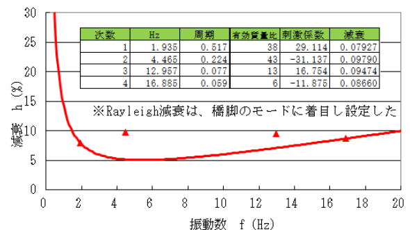
図-4 Rayleigh 減衰曲線
