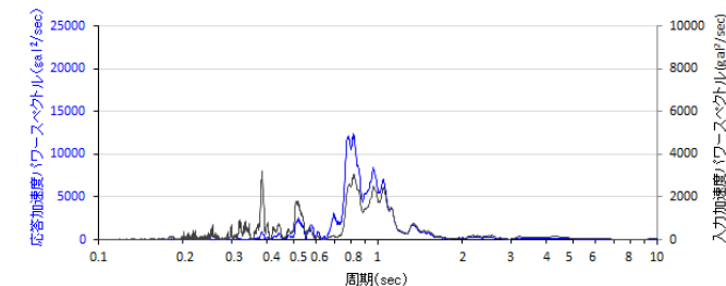
図-9 本震のパワースペクトル
