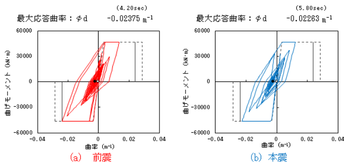
図-5 単独作用時の応答履歴曲線
