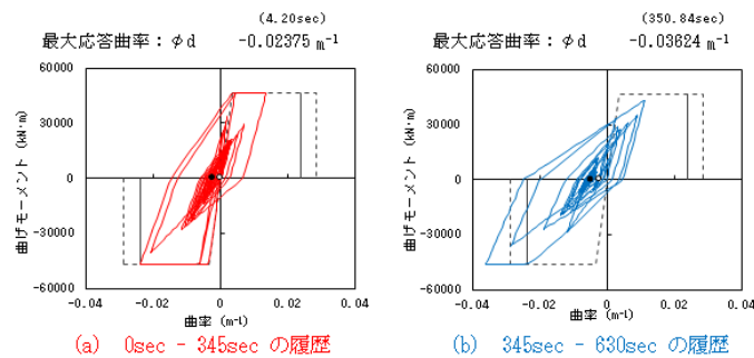
図-6 連続作用時の応答履歴曲線
