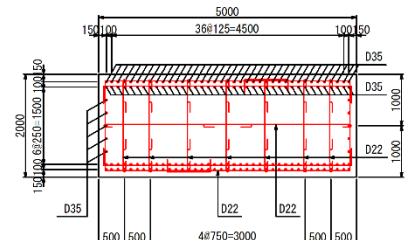
圖-3 橋脚柱基部断面圖
