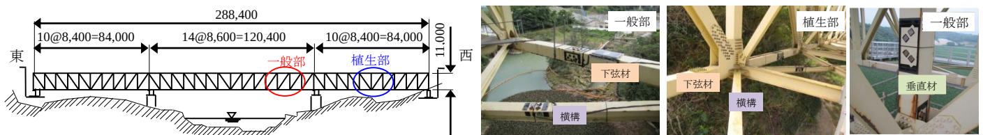
図 1 対象橋梁の諸元、および試験体の設置状況
