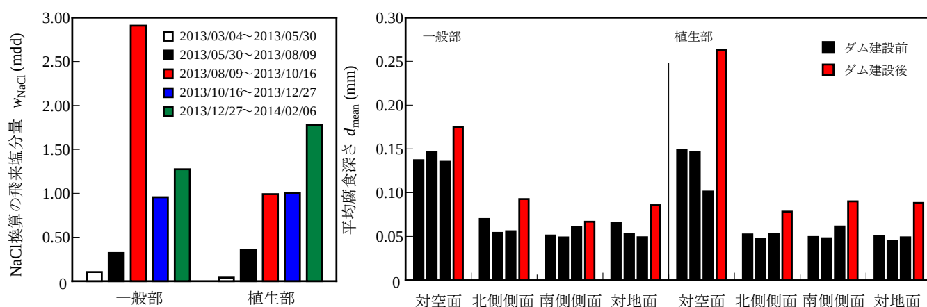
図4 ダム建設後における飛来塩分量 w_{NaCl}
