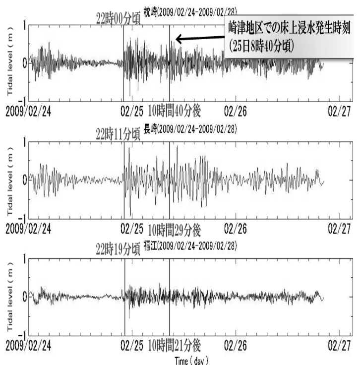
図-2 2009年2月24~27日の副振動の時系列
