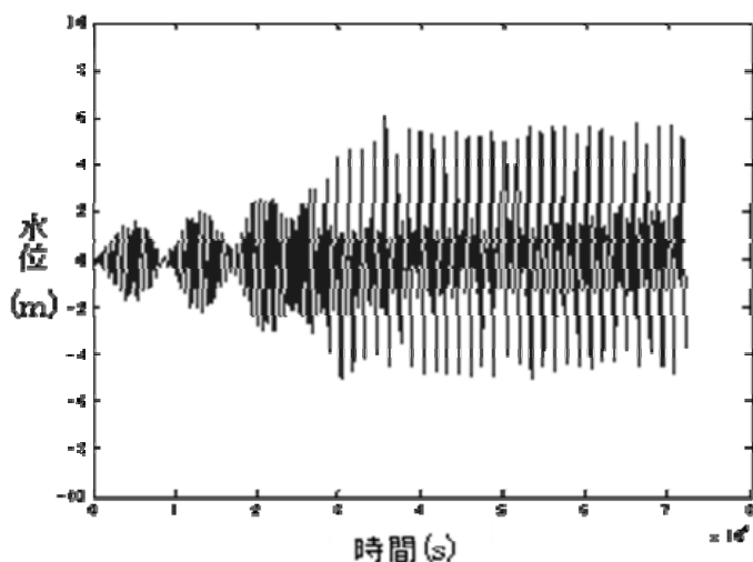
図-3 崎津湾中央部の水位の時系列（計算）
