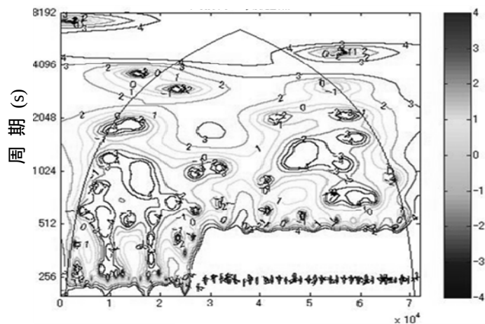
図-4 計算水位のウェーブレット変換結果
