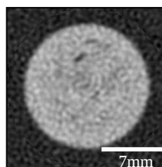
図 3. 円柱氷供試体の CT 画像
