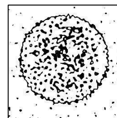
図 4. 二値化画像
