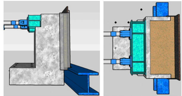
図-1 実験供試体概要図
