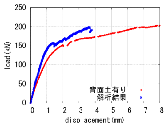
図-6 荷重-変位関係の比較
