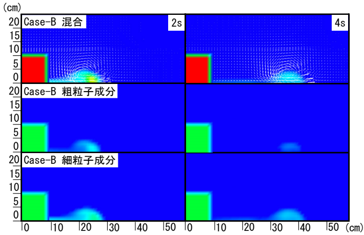
図-3 濁水塊の相対密度差コンターと流速ベクトル
