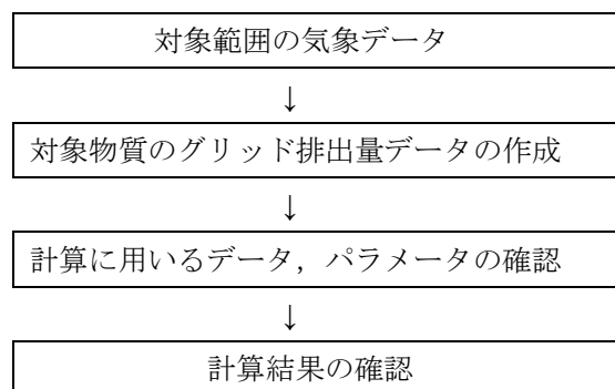
図1 解析手順
