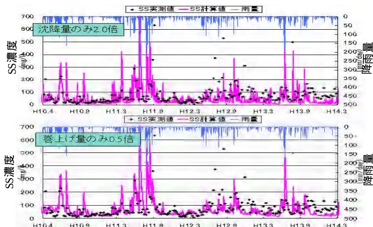
図-3 SS計算結果(底泥堆積量の増加を想定)
