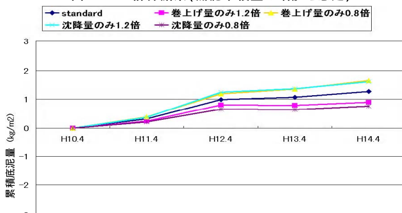
図-4 累積底泥量の経年変化
