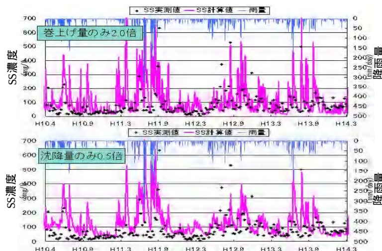
図-2 SS計算結果（底泥堆積量の減少を想定）
