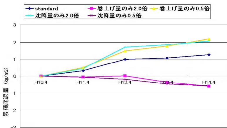
図-1 累積底泥量の経年変化
