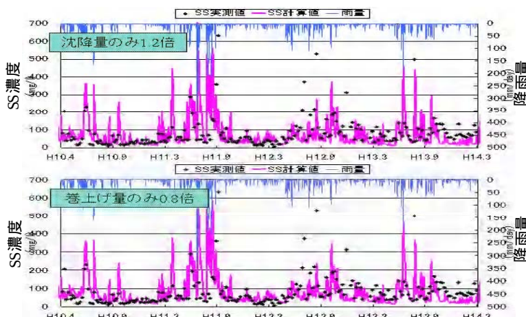
図-6 SS計算結果(底泥堆積量の増加を想定)
