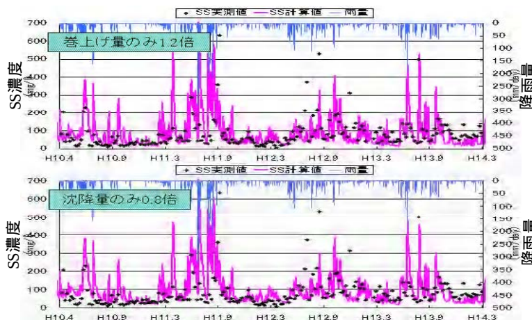
図-5 SS計算結果(底泥堆積量の減少を想定)
